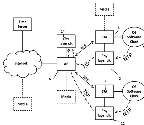
Multiple-protocol layer synchronisation technique
