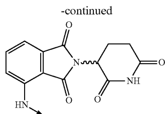
Pomalidomide
