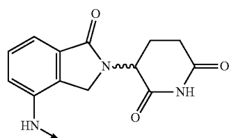
Lenalidomide
