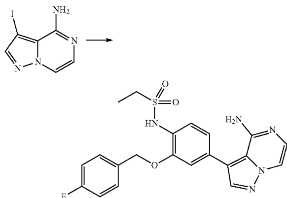
Step 1: N-(4-(4-Aminopyrazolo[1,5-a]pyrazin-3-yl)-2-((4-fluorophenyl)methoxy)phenyl)ethane-1-sulfonamide
