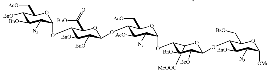
EDCBA Pentamer-CB C_{101}H_{105}N_9O_{30} Mol. Wt.: 1924.96
