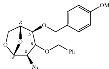
Monomer A-2
