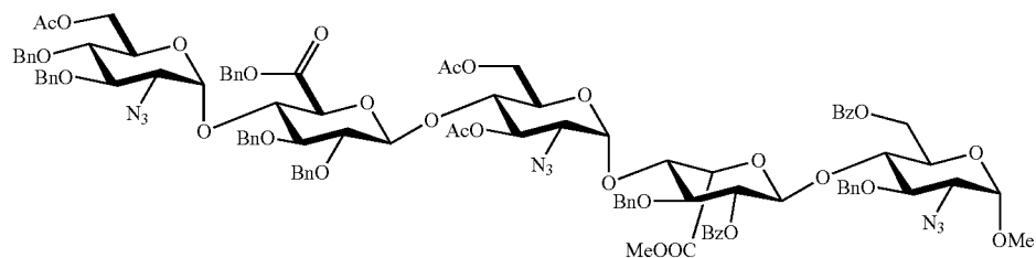
EDCBA Pentamer-CB
