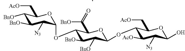
EDC-2-CB C_{57}H_{64}N_6O_{20} Mol. Wt.: 1153.15
