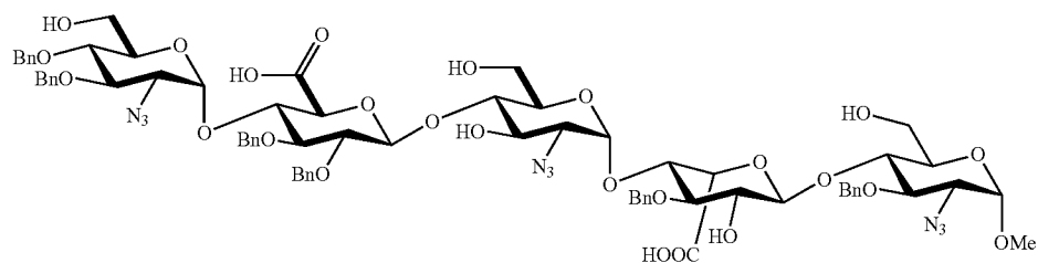
API-1-CB
