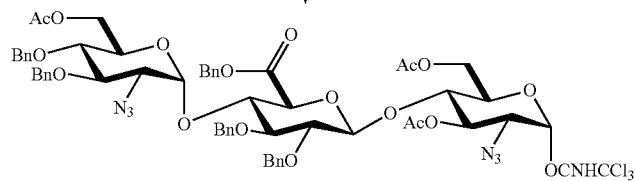
EDC-3-CB C_{61}H_{64}Cl_3N_7O_{18} Mol. Wt.: 1289.56
