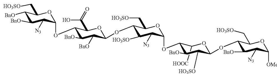
API-2-CB
