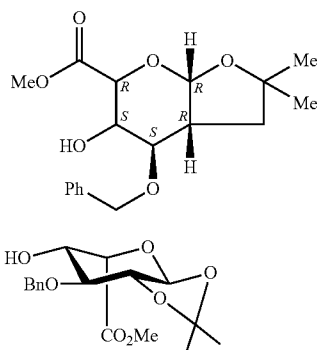
Monomer B-1
