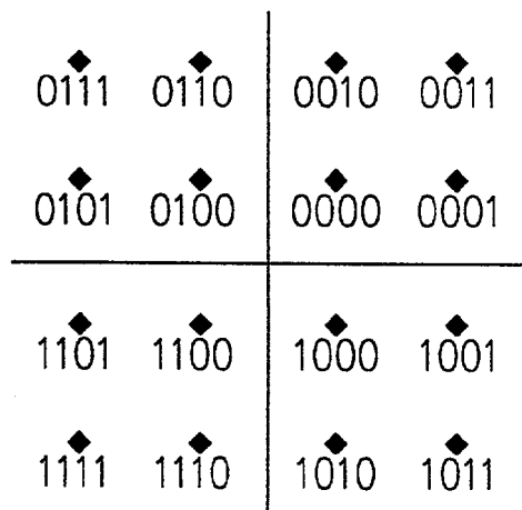
FIG. 12c 4 BITS PER BAUD
