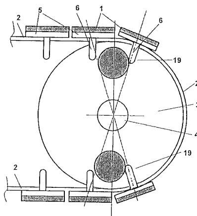
TEILSCHNITT B-B
