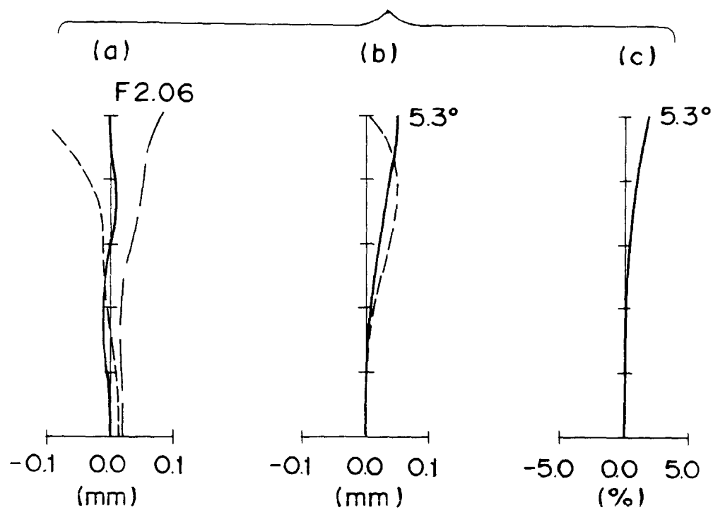
Fig. 7 ( f = 31.693 )
