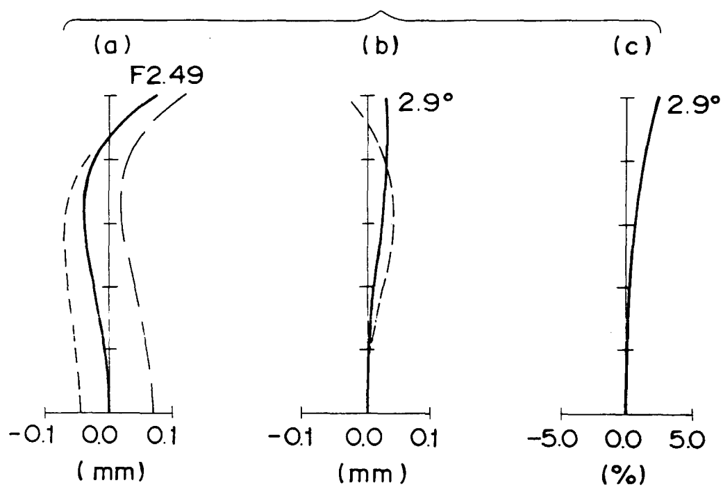
Fig. 11 ( f=59.832 )
