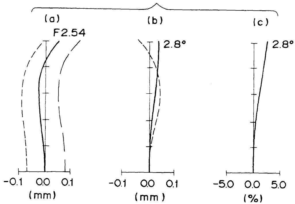
Fig. 8 ( f = 60.200 )
