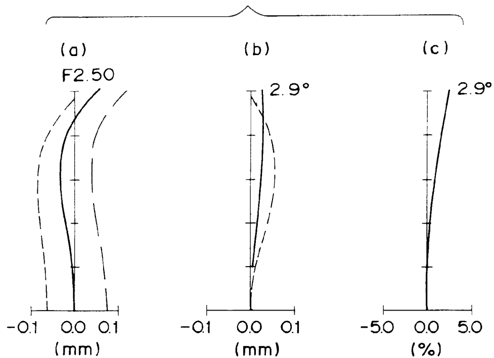
Fig. 5 ( f = 59.387 )
