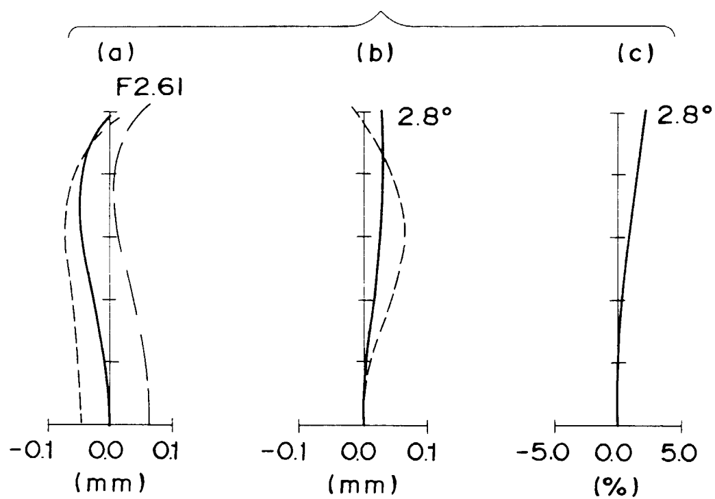
Fig. 15 ( f = 59.508 )
