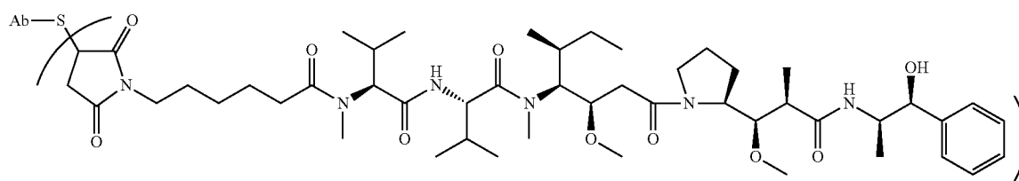
Ab-MC-MMAE
