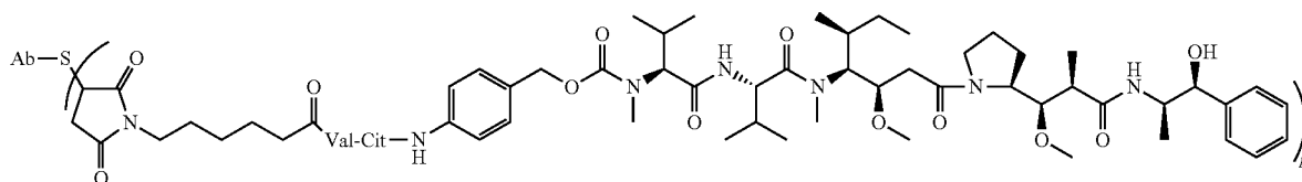
Ab-MC-vc-PAB-MMAE
