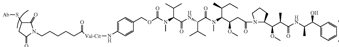
Ab-MC-vc-PAB-MMAE
