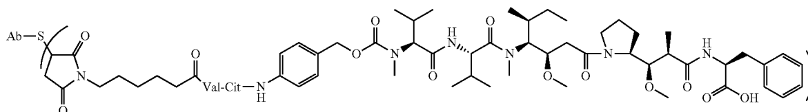
Ab-MC-vc-PAB-MMAF
