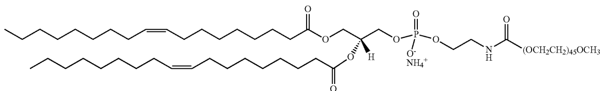
DOPE-PEG2000
