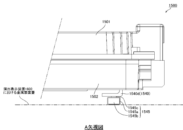
A矢視図
