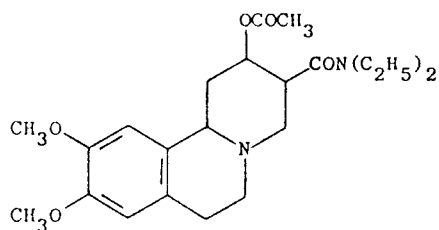
benzquinamide
