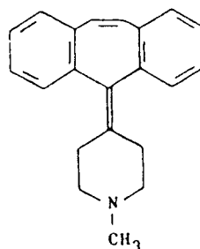
cypheptadine
