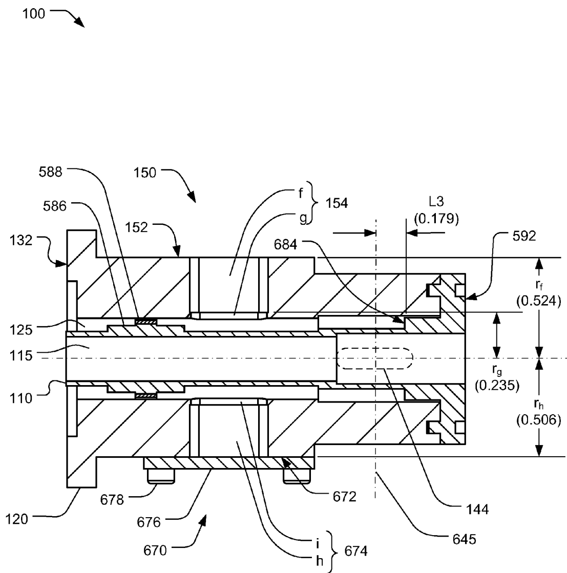
FIG. 6 Section B-B
