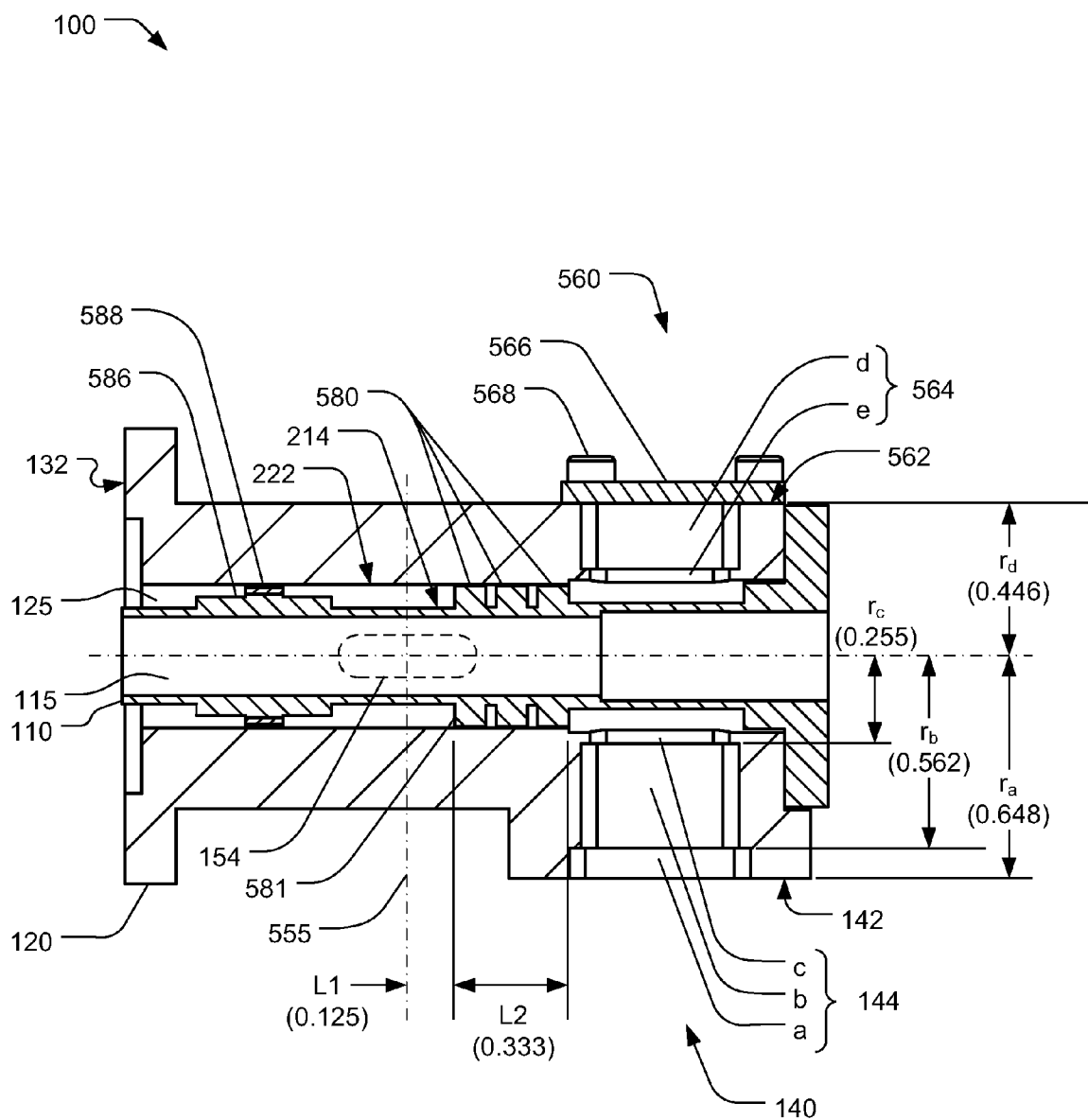
FIG. 5 Section A-A
