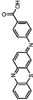
3-(4'-カルボキシフェニル)イミノ-3H-フエノチアジン エノチアジン
