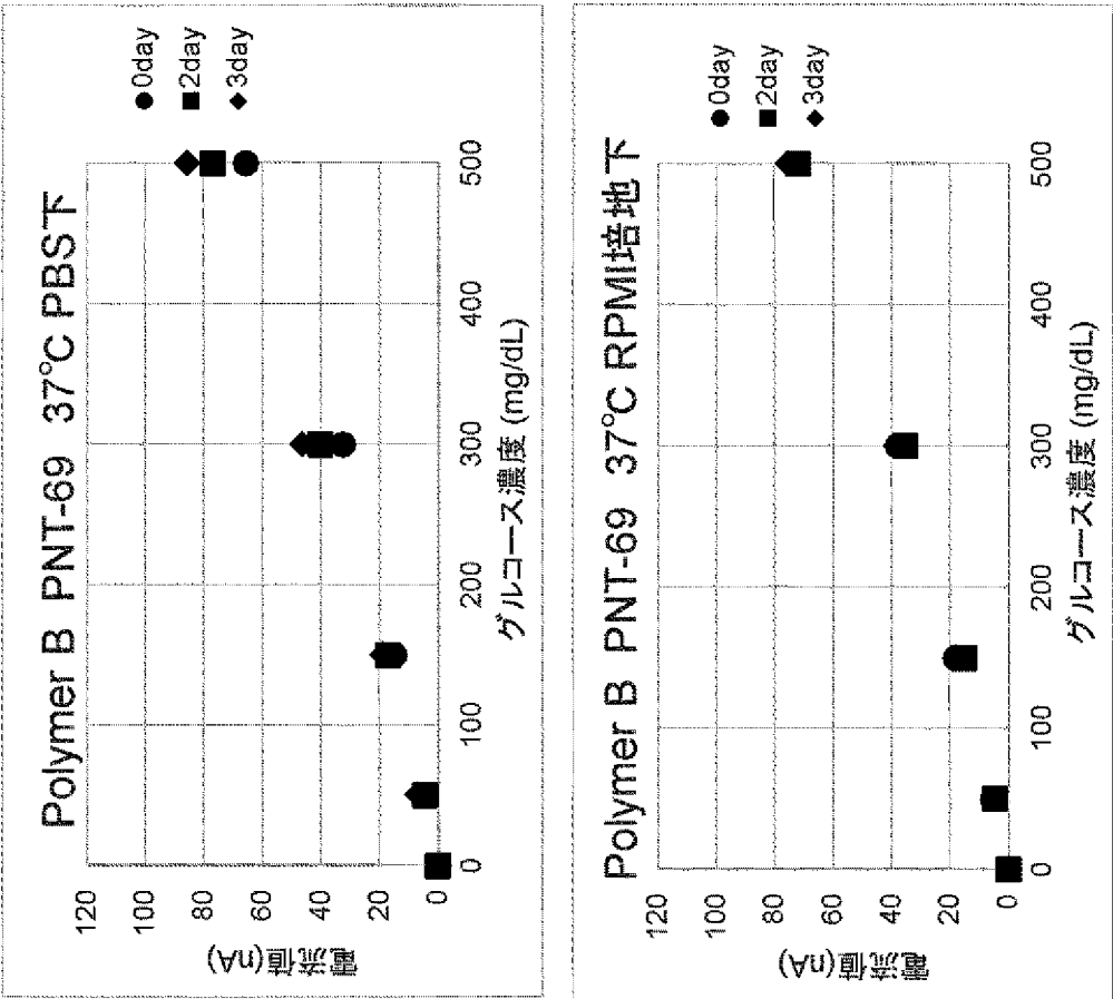
実施例3-3 (ポリマーB・PNT-69)
