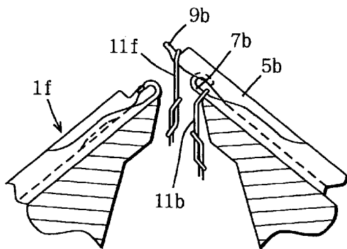
F I G. 2 - b
