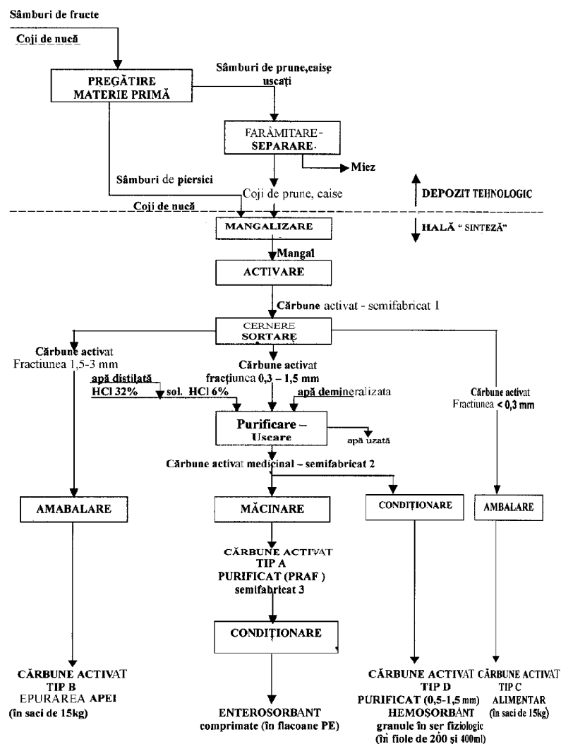
Schema fluxului tehnologic al procedurii de obținere a cărbunelui activat din sâmburi de fructe și coji de nuci
