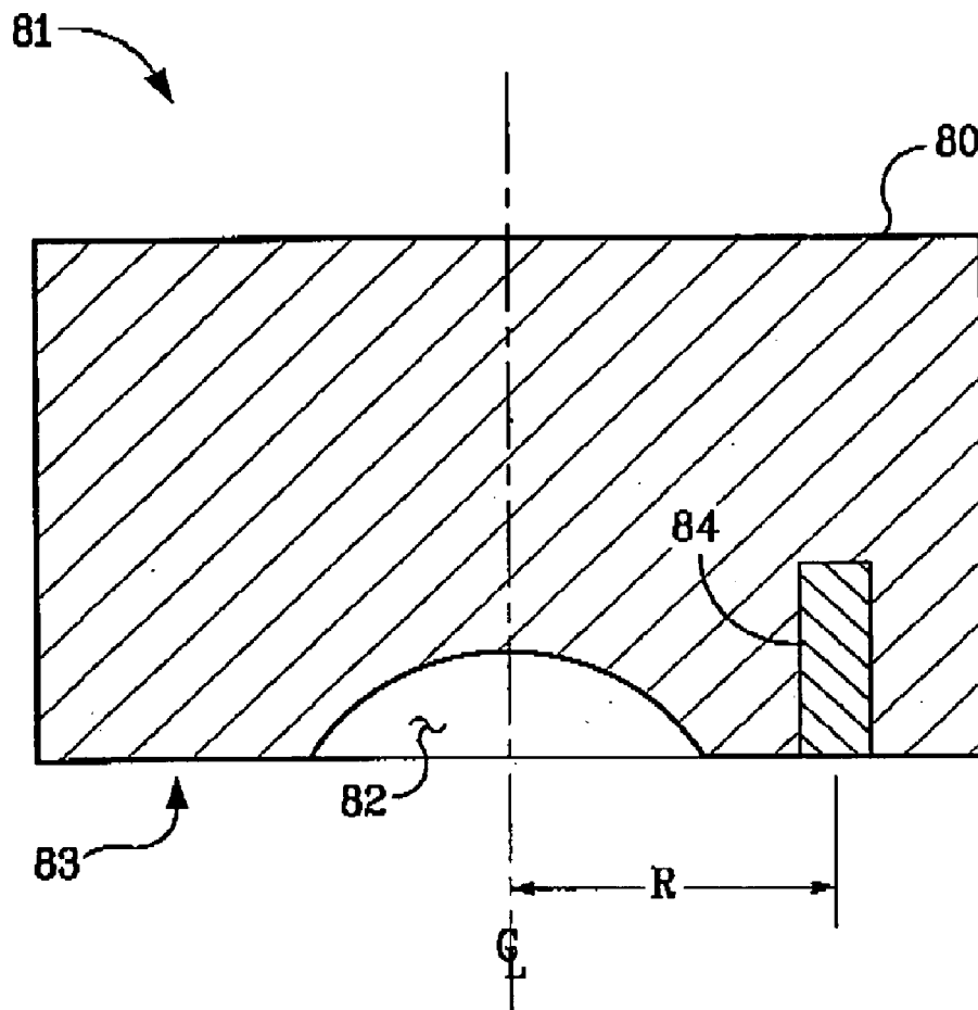
SEC A-A FIG. 9
