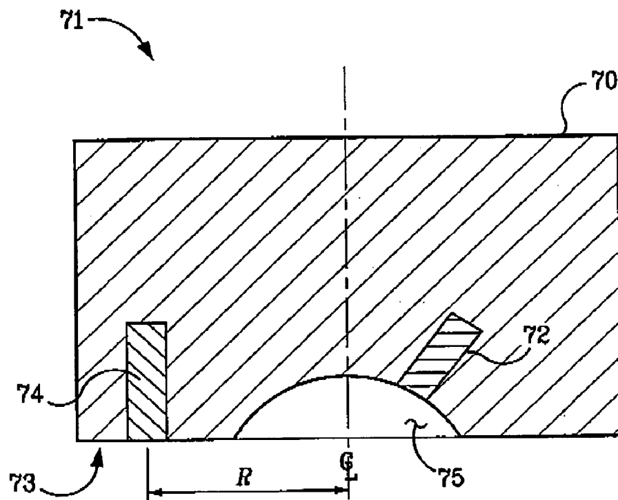
SEC A-A FIG. 8
