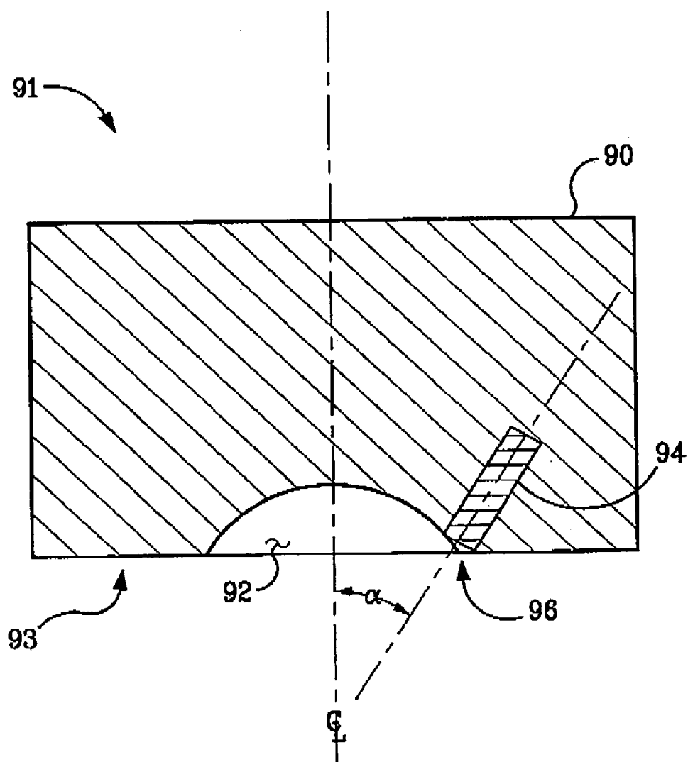
SEC A-A FIG. 10
