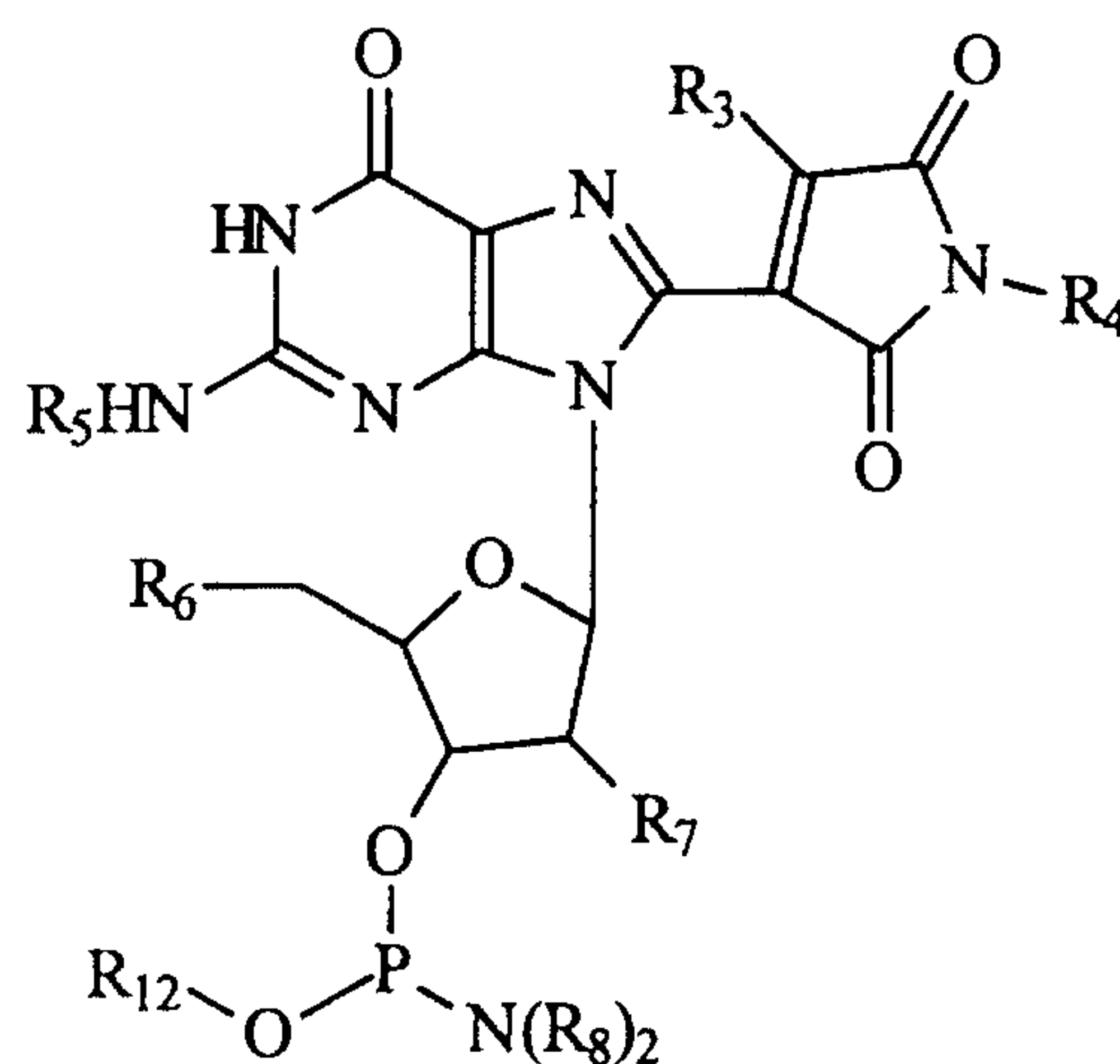
Structure Y
