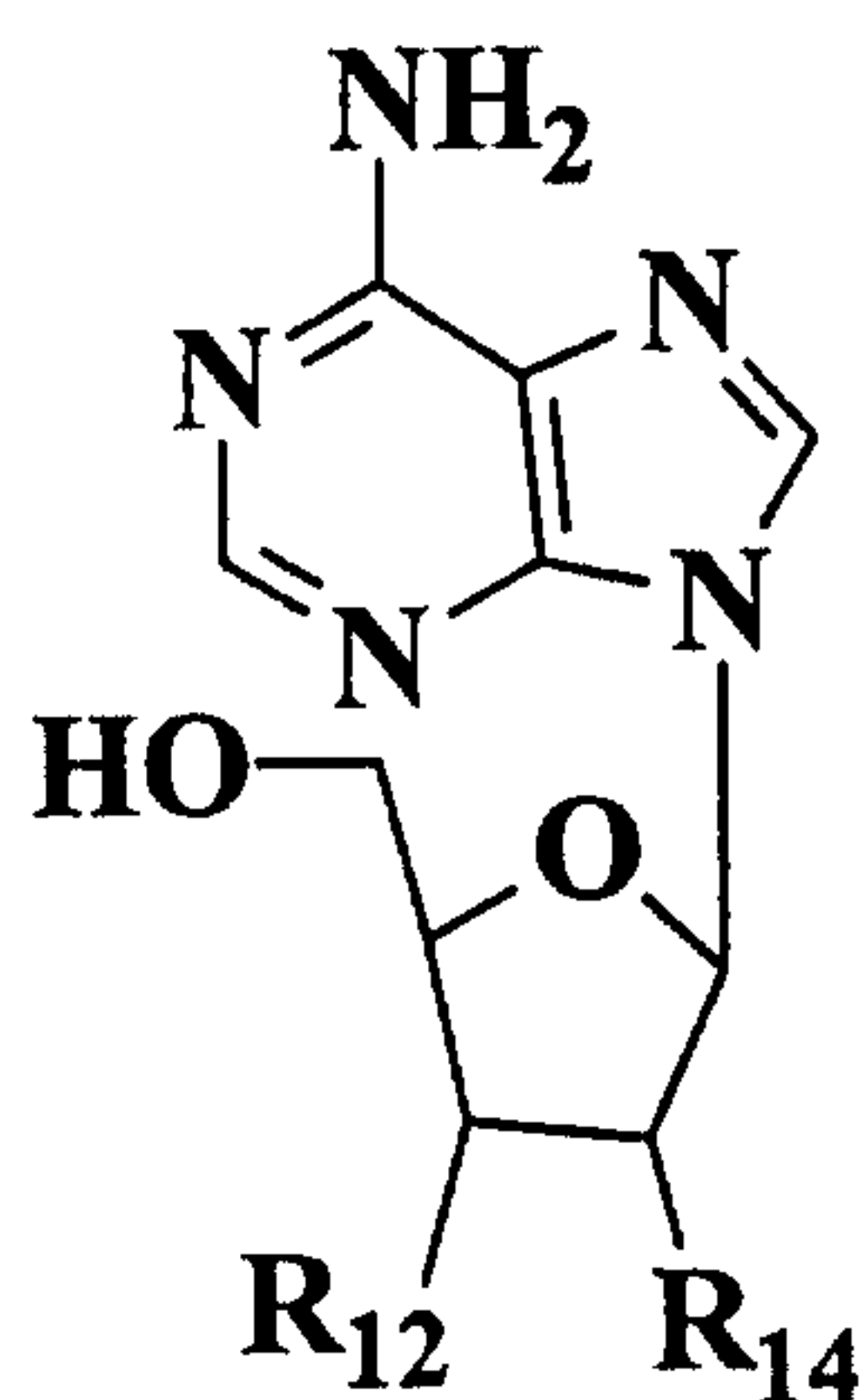
Adenosine
