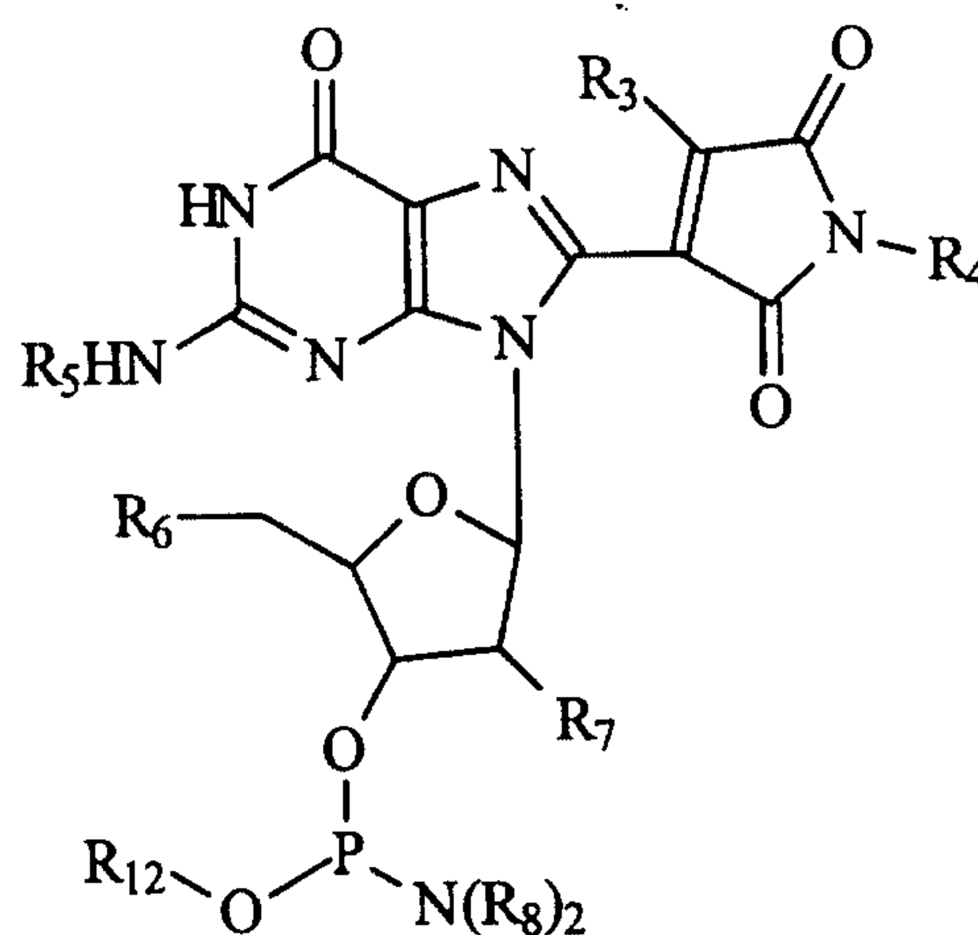
Structure Y
