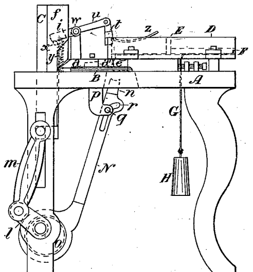
FIG. 2. SIDE ELEVATION
