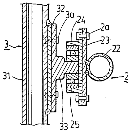
FIG. 4 (4-4')
