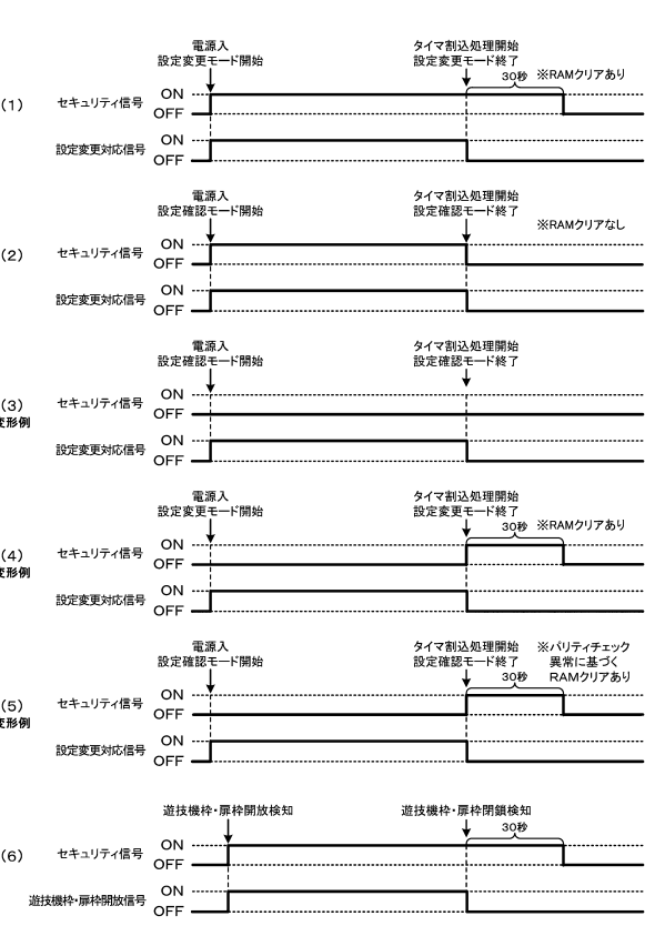
【図9-40】 セキュリティ信号及び設定変更対応信号の出力期間
