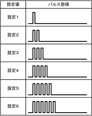
設定変更対応信号 (パルス態様)
