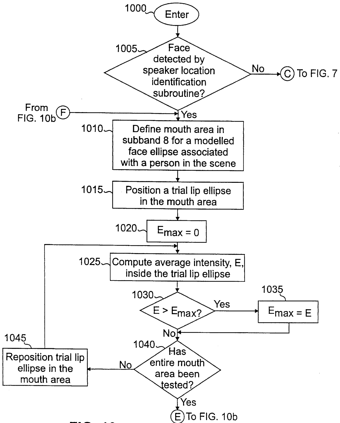
FIG. 10a
