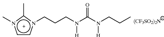
Acyclic amide IL 3
