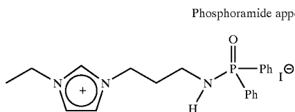
Phosphoramidate appended IL 1
