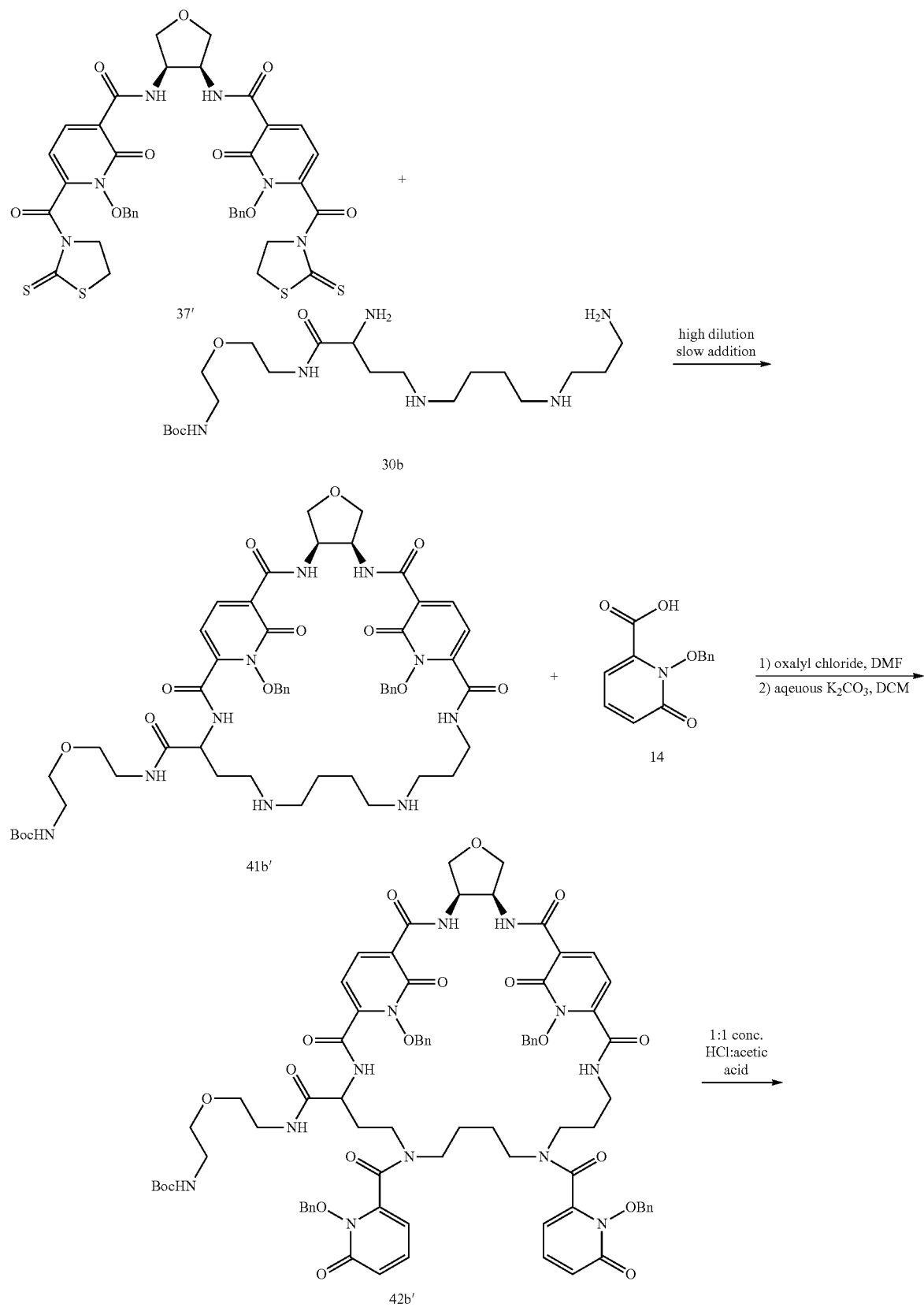
Scheme 16.
