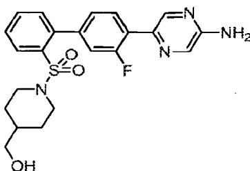
(1-([4'-(5-Aminopyrazin-2-yl)-3'-fluorobiphenyl-2-yl]sulfonyl)piperidin-4-yl)methanol
