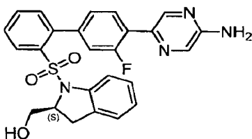
(S)-(1-([4'-(5-Aminopyrazin-2-yl)-3'-fluorobiphenyl-2-yl]sulfonyl)-2,3-dihydro-1H-indol-2-yl)-methanol
