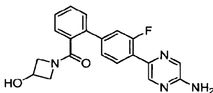
1-([4'-(5-Aminopyrazin-2-yl)-3'-fluorobiphenyl-2-yl]carbonyl)azetidin-3-ol
