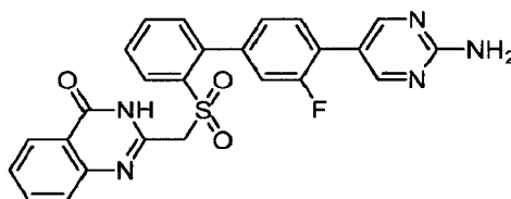
2-(((4'-(2-Aminopyrimidin-5-yl)-3'-fluoro-[1,1'-biphenyl]-2-yl)sulfonyl)methyl)quinazolin-4(3H)-one
