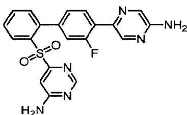
6-([4'-(5-Aminopyrazin-2-yl)-3'-fluorobiphenyl-2-yl]sulfonyl)pyrimidin-4-amine
