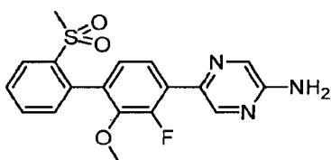
5-[3-Fluoro-2-methoxy-2'-(methylsulfonyl)biphenyl-4-yl]pyrazin-2-amine.
