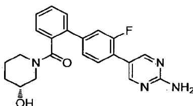
(3 R )-1-([4'-(2-Aminopyrimidin-5-yl)-3'-fluorobiphenyl-2-yl]carbonyl)piperidin-3-ol
