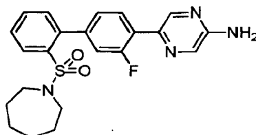
5-{2'-[(Azepan-1-yl)sulfonyl]-3-fluorobiphenyl-4-yl}pyrazin-2-amine
