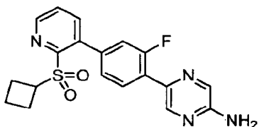
5-(4-(2-(Cyclobutylsulfonyl)pyridin-3-yl)-2-fluorophenyl)pyrazin-2-amine hydrochloride
