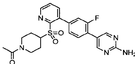
1-((3-(4-(2-Aminopyrimidin-5-yl)-3-fluorophenyl)pyridine-2-yl)sulfonyl)piperidin-1-yl)ethanone
