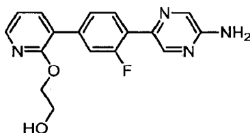
2-({3-[4-(5-Aminopyrazin-2-yl)-3-fluorophenyl]pyridin-2-yl}oxy)ethanol.
