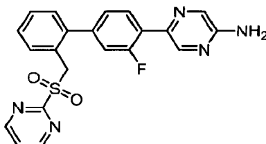
5-(3-Fluoro-2'--((pyrimidin-2-ylthio)methyl)biphenyl-4-yl)pyrazin-2-amine
