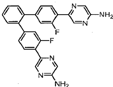
5,5'-(3,3'-Difluoro-1,1':2',1''-terphenyl-4,4''-diyl)dipyrazin-2-amine.
