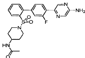
N -(1-([4'-(5-Aminopyrazin-2-yl)-3'-fluorobiphenyl-2-yl]sulfonyl)piperidin-4-yl)acetamide
