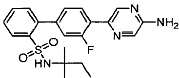
4'-(5-Aminopyrazin-2-yl)-N-(1,1-dimethylpropyl)-3'-fluorobiphenyl-2-sulfonamide
