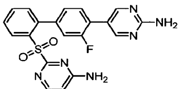
5-{2'-[(4-aminopyrimidin-2-yl)sulfonyl]-3-fluorobiphenyl-4-yl}pyrimidin-2-amine
