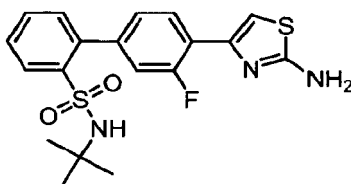
4'-(2-Amino-1,3-thiazol-4-yl)- N -tert-butyl-3'-fluorobiphenyl-2-sulfonamide
