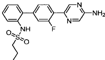
N -[4'-(5-Aminopyrazin-2-yl)-3'-fluorobiphenyl-2-yl]propane-1-sulfonamide
