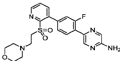
5-(2-Fluoro-4-(2-((2-morpholinoethyl)sulfonyl)pyridine-3-yl)phenyl)pyrazin-2-amine
