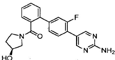
(3S)-1-([4'-(2-Aminopyrimidin-5-yl)-3'-fluorobiphenyl-2-yl]carbonyl)pyrrolidin-3-ol
