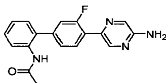
N-[4'-(5-Aminopyrazin-2-yl)-3'-fluorobiphenyl-2-yl]acetamide
