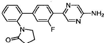
1-[4'-(5-Aminopyrazin-2-yl)-3'-fluorobiphenyl-2-yl]pyrrolidin-2-one
