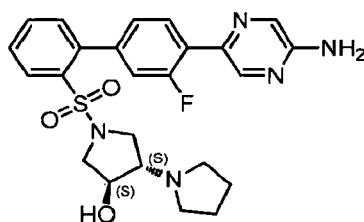
Racemic-1'-([4'-(5-Aminopyrazin-2-yl)-3'-fluorobiphenyl-2-yl]sulfonyl)-1,3'-bipyrrolidin-4'-ol
