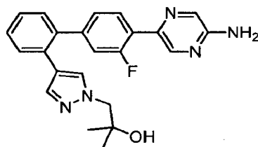
1-{4-[4'-(5-Aminopyrazin-2-yl)-3'-fluorobiphenyl-2-yl]-1H-pyrazol-1-yl}-2-methylpropan-2-ol.
