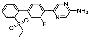
5-[2'-(Ethylsulfonyl)-3-fluorobiphenyl-4-yl]pyrazin-2-amine
