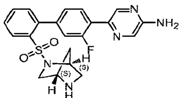
5-(2'-((1 S ,4 S )-2,5-Diazabicyclo[2.2.1]heptan-2-ylsulfonyl)-3-fluoro-[1,1'-biphenyl]-4-yl)pyrazin-2-amine
