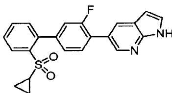
5-[2'-(Cyclopropylsulfonyl)-3-fluorobiphenyl-4-yl]-1H-pyrrolo[2,3-b]pyridine
