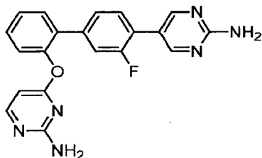
4-([4'-(2-Aminopyrimidin-5-yl)-3'-fluorobiphenyl-2-yl]oxy)pyrimidin-2-amine
