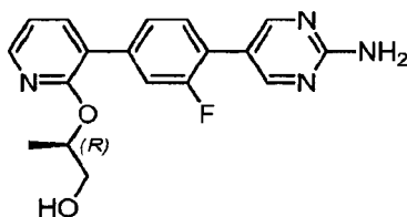
(2I)-2-({3-[4-(2-Aminopyrimidin-5-yl)-3-fluorophenyl]pyridin-2-yl}oxy)propan-1-ol.
