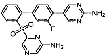
5-{2'-[(6-Aminopyrazin-2-yl)sulfonyl]-3-fluorobiphenyl-4-yl}pyrimidin-2-amine
