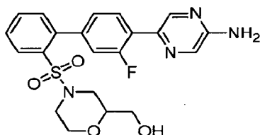
racemic (4'-((5-Aminopyrazin-2-yl)-3'-fluorobiphenyl-2-yl)sulfonyl)morpholin-2-yl)methanol
