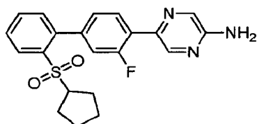
5-{2'-(Cyclopentylsulfonyl)-3-fluorobiphenyl-4-yl}pyrazin-2-amine
