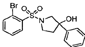
1-((2-Bromophenyl)sulfonyl)-3-phenylpyrrolidin-3-ol.
