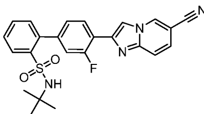
N -tert-Butyl-4'-(6-cyanoimidazo[1,2-a]pyridin-2-yl)-3'-fluorobiphenyl-2-sulfonamide
