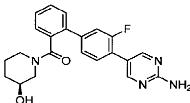
(3S)-1-([4'-(2-Aminopyrimidin-5-yl)-3'-fluorobiphenyl-2-yl]carbonyl)piperidin-3-ol
