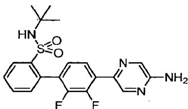
4'-(5-Aminopyrazin-2-yl)-N-tert-butyl-2',3'-difluorobiphenyl-2-sulfonamide
