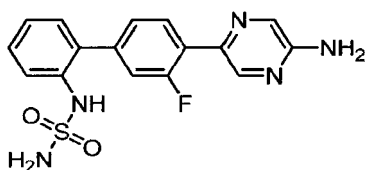
N -[4'-(5-Aminopyrazin-2-yl)-3'-fluorobiphenyl-2-yl]sulfamide
