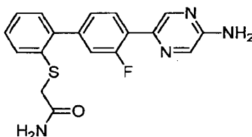
2-([4'-(5-Aminopyrazin-2-yl)-3'-fluorobiphenyl-2-yl]sulfanyl)acetamide
