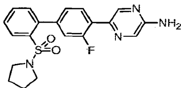
5-[3-fluoro-2'-(pyrrolidin-1-ylsulfonyl)biphenyl-4-yl]pyrazin-2-amine
