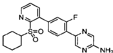
5-(4-(2-(Cyclohexylsulfonyl)pyridin-3-yl)-2-fluorophenyl)pyrazin-2-amine hydrochloride
