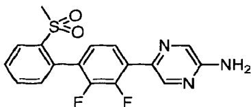
5-[2,3-Difluoro-2'-(methylsulfonyl)biphenyl-4-yl]pyrazin-2-amine
