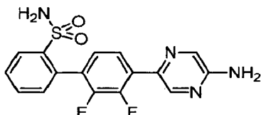
4'-(5-Aminopyrazin-2-yl)-2',3'-difluorobiphenyl-2-sulfonamide
