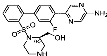
(R)-(1-((4'-(5-Aminopyrazin-2-yl)-3'-fluoro-[1,1'-biphenyl]-2-yl)sulfonyl)piperazin-2-yl)methanol
