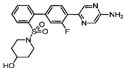
1-([4'-(5-Aminopyrazin-2-yl)-3'-fluorobiphenyl-2-yl]sulfonyl)piperidin-4-ol
