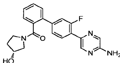
(3 R )-1-([4'-(5-Aminopyrazin-2-yl)-3'-fluorobiphenyl-2-yl]carbonyl)pyrrolidin-3-ol
