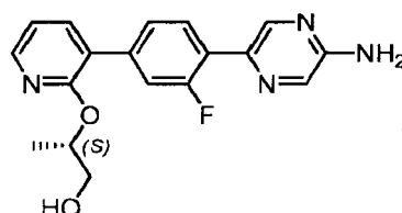
(2R)-2-({3-[4-{5-Aminopyrazin-2-yl}-3-fluorophenyl]pyridin-2-yl}oxy)propan-1-ol.
