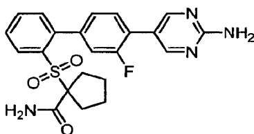
1-([4'-(2-Aminopyrimidin-5-yl)-3'-fluorobiphenyl-2-yl]sulfonyl)cyclopentanecarboxamide
