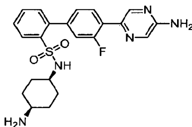
cis -N-(4-Aminocyclohexyl)-4'-(5-aminopyrazin-2-yl)-3'-fluorobiphenyl-2-sulfonamide
