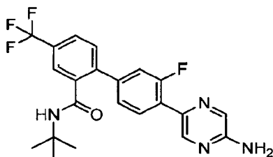
2-[4-(5-Aminopyrazin-2-yl)-3-fluoro-phenyl]-N-tert-butyl-5-(trifluoromethyl)benzamide
