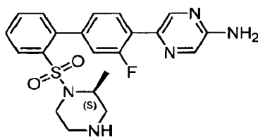
(S)-5-(3-Fluoro-2'-((2-methylpiperazin-1-yl)sulfonyl)-[1,1'-biphenyl]-4-yl)pyrazin-2-amine
