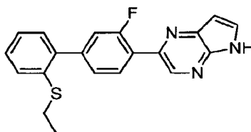
2-[2'-(Ethylsulfanyl)-3-fluorobiphenyl-4-yl]-5H-pyrrolo[2,3-b]pyrazine
