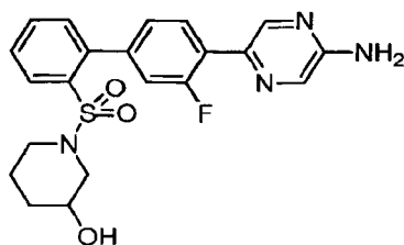
racemic 1-([4'-(5-Aminopyrazin-2-yl)-3'-fluorobiphenyl-2-yl]sulfonyl)piperidin-3-ol
