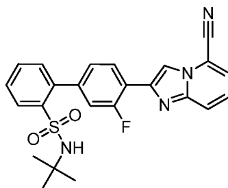
N -tert-Butyl-4'-(5-cyanoimidazo[1,2-a]pyridin-2-yl)-3'-fluorobiphenyl-2-sulfonamide
