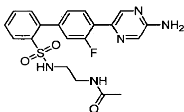
N -[2-({[4'-(5-Aminopyrazin-2-yl)-3'-fluorobiphenyl-2-yl]sulfonyl}amino)ethyl]acetamide
