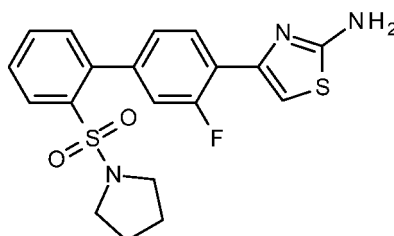
4-[3-Fluoro-2'-(pyrrolidin-1-ylsulfonyl)biphenyl-4-yl]-1,3-thiazol-2-amine
