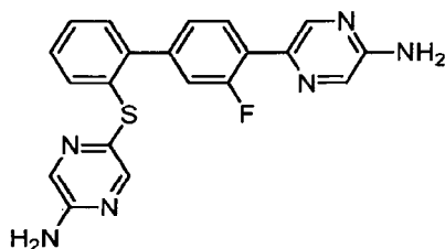
5-([4'-(5-Aminopyrazin-2-yl)-3'-fluorobiphenyl-2-yl]sulfanyl)pyrazin-2-amine
