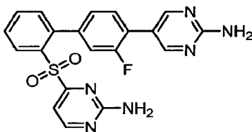
4-{[4'-(2-Aminopyrimidin-5-yl)-3'-fluorobiphenyl-2-yl]sulfonyl}pyrimidin-2-amine
