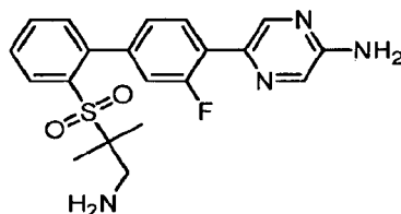
5-{2'-[(2-Amino-1,1-dimethylethyl)sulfonyl]-3-fluorobiphenyl-4-yl}pyrazin-2-amine
