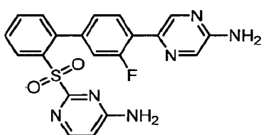
2-([4'-(5-Aminopyrazin-2-yl)-3'-fluorobiphenyl-2-yl]sulfonyl)pyrimidin-4-amine
