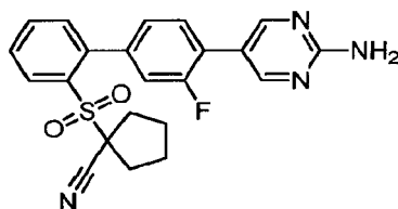
1-([4'-(2-Aminopyrimidin-5-yl)-3'-fluorobiphenyl-2-yl]sulfonyl)cyclopentanecarbonitrile
