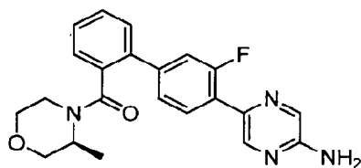
5-(3-Fluoro-2'--[(3S)-3-methylmorpholin-4-yl]carbonyl)biphenyl-4-yl)pyrazin-2-amine
