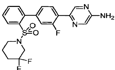
5-{2'-[(3,3-Difluoropiperidin-1-yl)sulfonyl]-3-fluorobiphenyl-4-yl}pyrazin-2-amine
