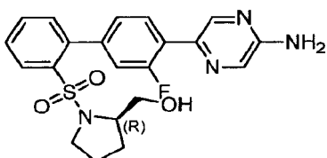
(R)-1-((4'-((5-Aminopyrazin-2-yl)-3'-fluoro-[1,1'-biphenyl]-2-yl)sulfonyl)pyrrolidin-2-yl)methanol
