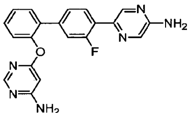
6-([4'-(5-Aminopyrazin-2-yl)-3'-fluorobiphenyl-2-yl]oxy)pyrimidin-4-amine
