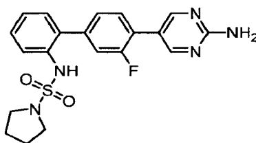
N -{[4'-(2-Aminopyrimidin-5-yl)-3'-fluorobiphenyl-2-yl]pyrrolidine-1-sulfonamide}
