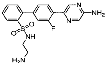
N -(2-Aminoethyl)-4'-({5-aminopyrazin-2-yl})-3'-fluorobiphenyl-2-sulfonamide
