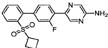
5-[2'-(Cyclobutylsulfonyl)-3-fluorobiphenyl-4-yl]pyrazin-2-amine
