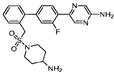
5-(2'-((4-Aminopiperidin-1-yl)sulfonyl)methyl)-3-fluorobiphenyl-4-ylpyrazin-2-amine hydrochloride
