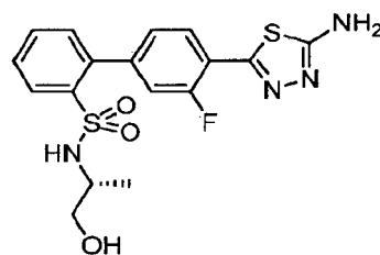
( R )-4'-((5-Amino-1,3,4-thiadiazol-2-yl)-3'-fluoro- N -(1-hydroxypropan-2-yl)-[1,1'-biphenyl]-2-sulfonamide
