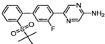
5-{2'-( tert -Butylsulfonyl)-3-fluorobiphenyl-4-yl}pyrazin-2-amine
