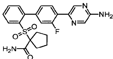
1-([4'-(5-Aminopyrazin-2-yl)-3'-fluorobiphenyl-2-yl]sulfonyl)cyclopentanecarboxamide
