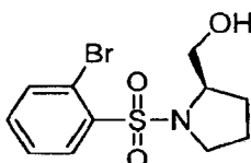
(R)-1-((2-Bromophenyl)sulfonyl)pyrrolidin-2-ylmethanol.
