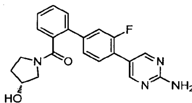
(3 R )-1-([4'-(2-Aminopyrimidin-5-yl)-3'-fluorobiphenyl-2-yl]carbonyl)pyrrolidin-3-ol
