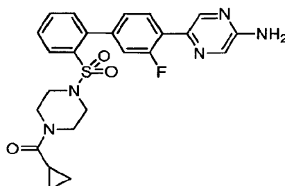
5-{2'-[4-(Cyclopropylcarbonyl)piperazin-1-yl)sulfonyl]-3-fluorobiphenyl-4-yl}pyrazin-2-amine
