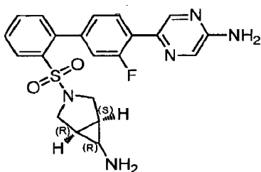
endo-3-((4'-((5-Aminopyrazin-2-yl)-3'-fluoro-[1,1'-biphenyl]-2-yl)sulfonyl)-3-azabicyclo[3.1.0]hexan-6-amine
