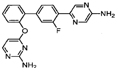
4-([4'-(5-Aminopyrazin-2-yl)-3'-fluorobiphenyl-2-yl]oxy)pyrimidin-2-amine
