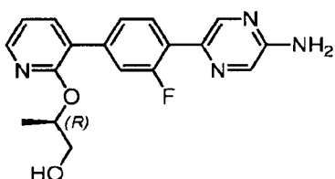
(2S)-2-({3-[4-(5-Aminopyrazin-2-yl)-3-fluorophenyl]pyridin-2-yl}oxy)propan-1-ol.
