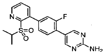
5-(2-Fluoro-4-((1-methylethyl)sulfonyl)pyridin-3-yl)phenyl)pyrimidin-2-amine
