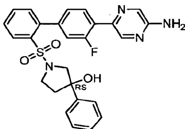
racemic 1-([4'-(5-Aminopyrazin-2-yl)-3'-fluorobiphenyl-2-yl]sulfonyl)-3-phenylpyrrolidin-3-ol
