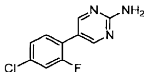
5-(4-Chloro-2-fluorophenyl)pyrimidin-2-amine
