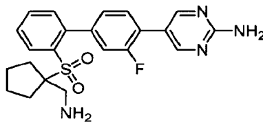
5-(2'-([1-(Aminomethyl)cyclopentyl]sulfonyl)-3-fluorobiphenyl-4-yl)pyrimidin-2-amine
