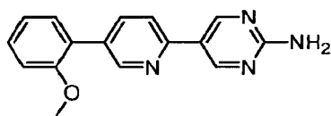
5-[5-(2-Methoxyphenyl)pyridin-2-yl]pyrimidin-2-amine.
