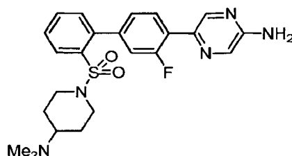
5-(2'-[4-(Dimethylamino)piperidin-1-yl]sulfonyl)-3-fluorobiphenyl-4-yl)pyrazin-2-amine
