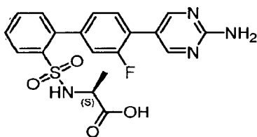
N -{[4'-(2-Aminopyrimidin-5-yl)-3'-fluorobiphenyl-2-yl]sulfonyl}-L-alanine
