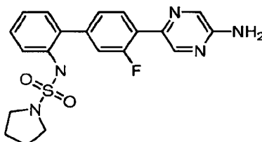
N-[4'-(5-Aminopyrazin-2-yl)-3'-fluorobiphenyl-2-yl]pyrrolidine-1-sulfonamide
