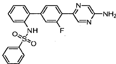
N -[4'-(5-Aminopyrazin-2-yl)-3'-fluorobiphenyl-2-yl]benzenesulfonamide
