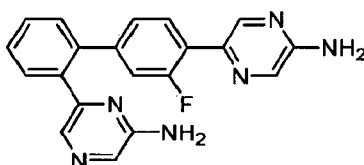
5-[2'-(6-Aminopyrazin-2-yl)-3-fluorobiphenyl-4-yl]pyrazin-2-amine.
