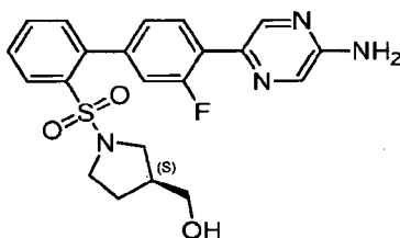
(S) -(1-((4'-(5-Aminopyrazin-2-yl)-3'-fluorobiphenyl-2-yl)sulfonyl)pyrrolidin-3-yl)methanol
