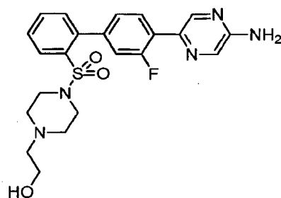
2-(4-([4'-(5-Aminopyrazin-2-yl)-3'-fluorobiphenyl-2-yl]sulfonyl)piperazin-1-yl)ethanol
