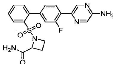
Racemic 1-([4'-(5-Aminopyrazin-2-yl)-3'-fluorobiphenyl-2-yl]sulfonyl)azetidine-2-carboxamide
