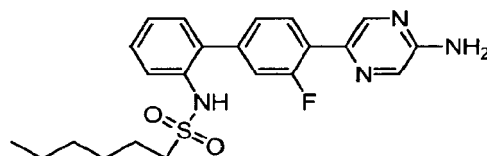
N -[4'-(5-Aminopyrazin-2-yl)-3'-fluorobiphenyl-2-yl]hexane-1-sulfonamide
