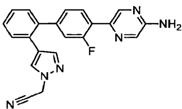
{4-[4'-(5-Aminopyrazin-2-yl)-3'-fluorobiphenyl-2-yl]-1 H -pyrazol-1-yl}acetonitrile.
