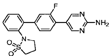
5-[2'-(1,1-Dioxidoisothiazolidin-2-yl)-3-fluorobiphenyl-4-yl]pyrimidin-2-amine
