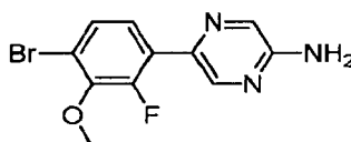
5-(4-Bromo-2-fluoro-3-methoxyphenyl)pyrazin-2-amine.
