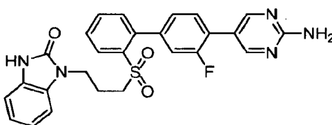
1-(3-(((4'-(2-Aminopyrimidin-5-yl)-3'-fluoro-[1,1'-biphenyl]-2-yl)sulfonyl)propyl)-1H-benzo[d]imidazol-2(3H)-one
