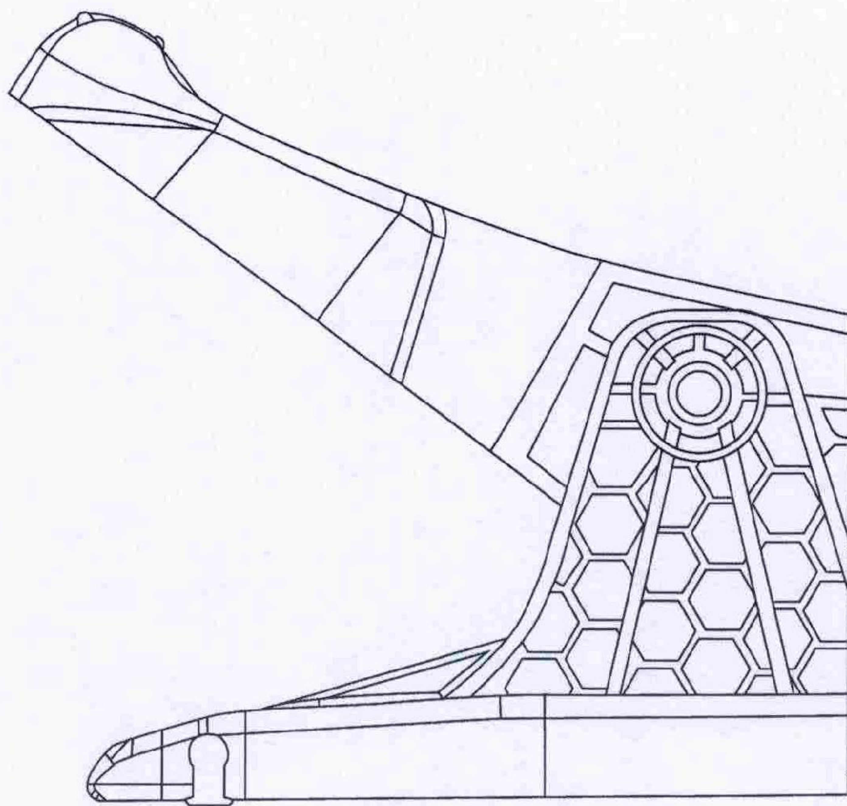
前視圖
