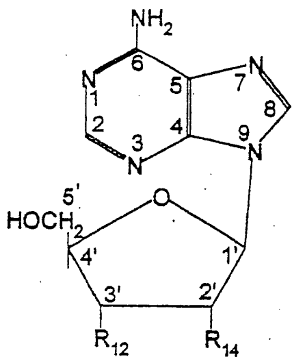
Adenosine
