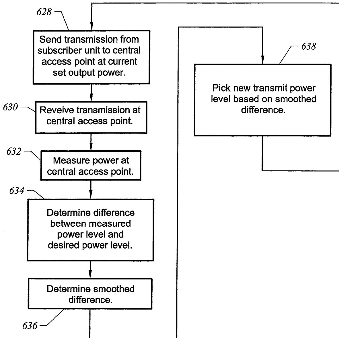
FIG. 6B
