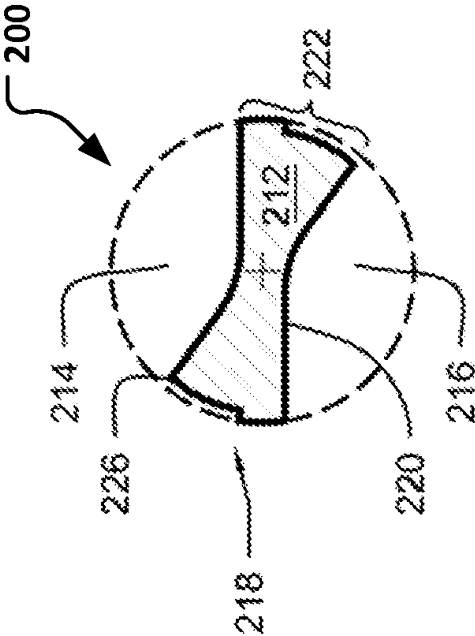
Section A-A
