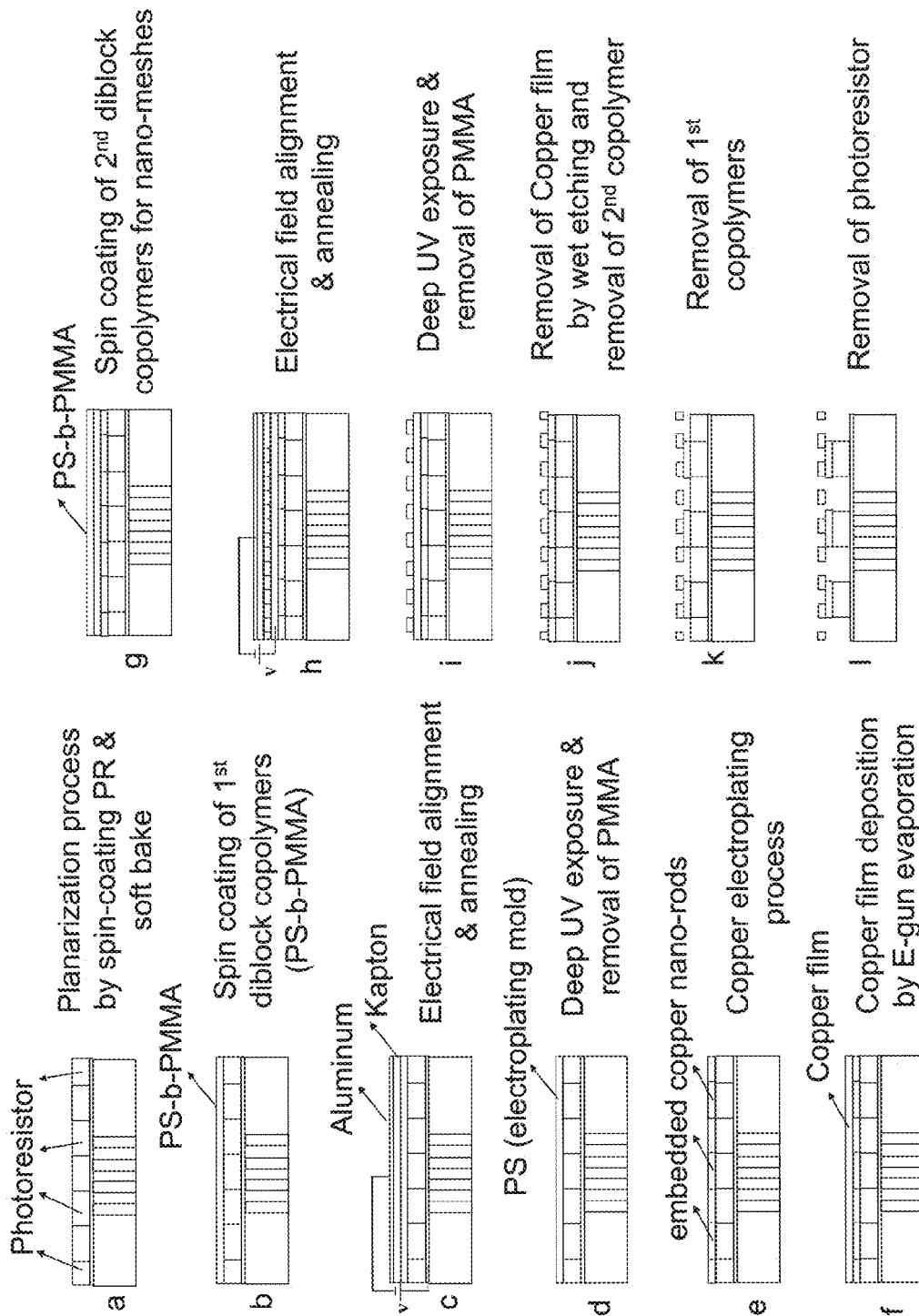
FIG. 19A
