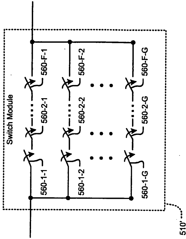
FIG. 19B
