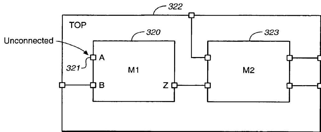
FIG. 35A : RTL code
