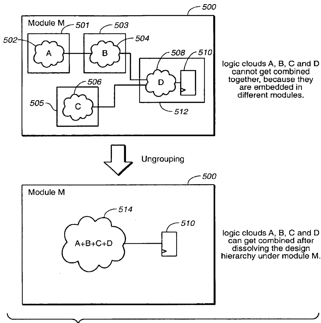
FIG. 22 : Hierarchy ungrouping.
