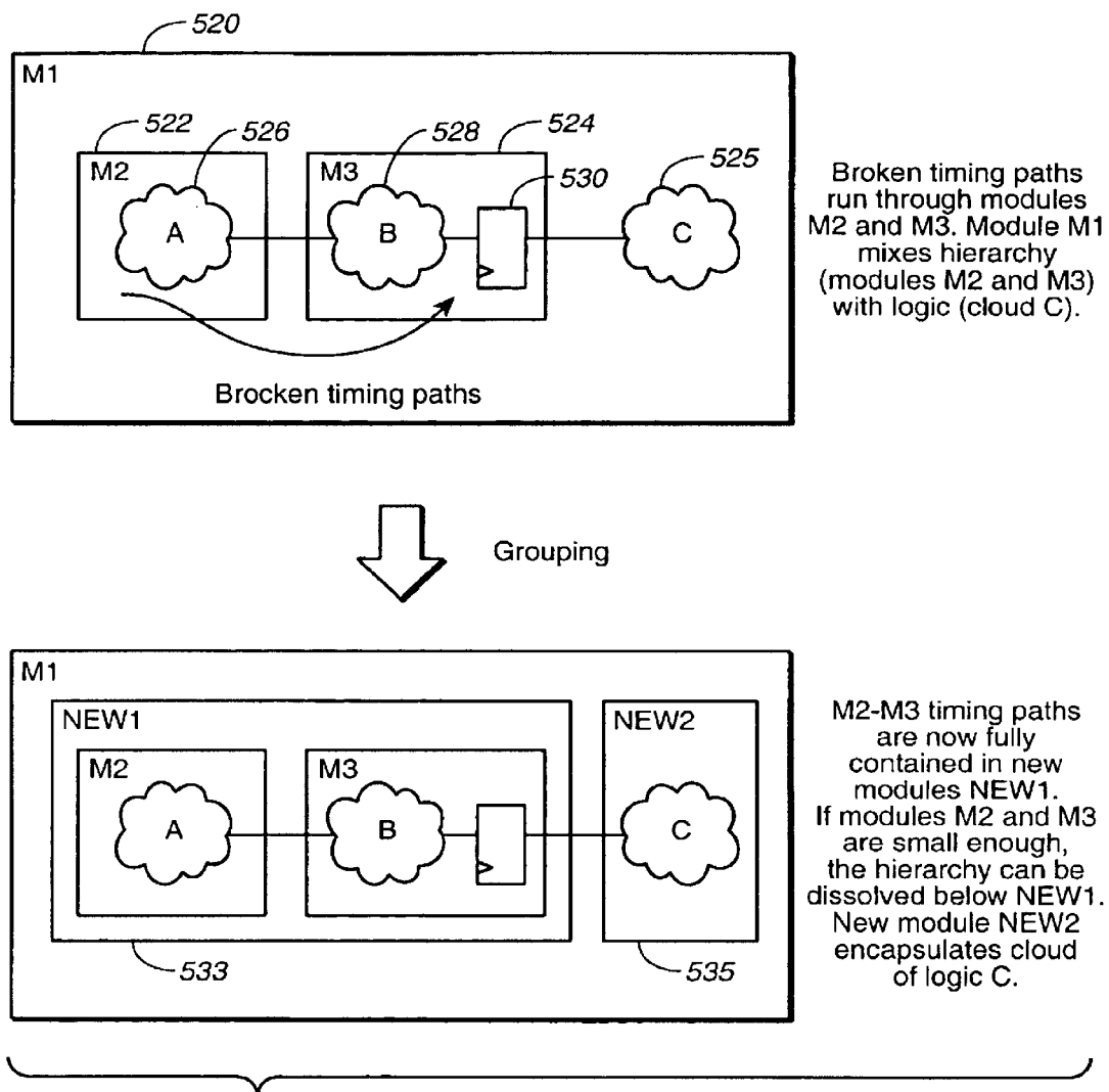
FIG. 23 : Hierarchy grouping.
