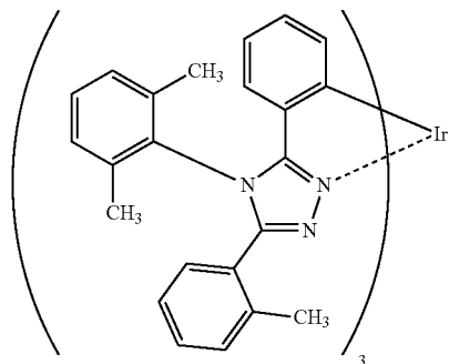
[Ir(mpptz-dmp) 3 ]
