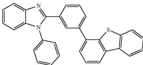
mDBTBlm-II
