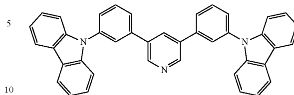
35DCzPPy
