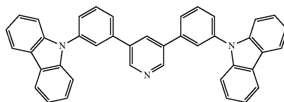
35DCzPPy
