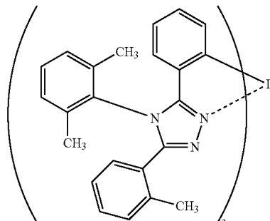
[Ir(mpptz-dmp) 3 ]
