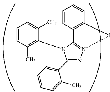
[Ir(mpptz-dmp) 3 ]
