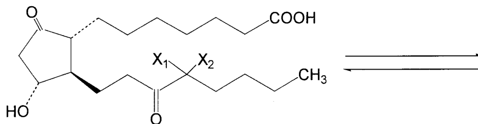
Tautomer I
