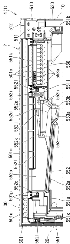
B-B断面図
