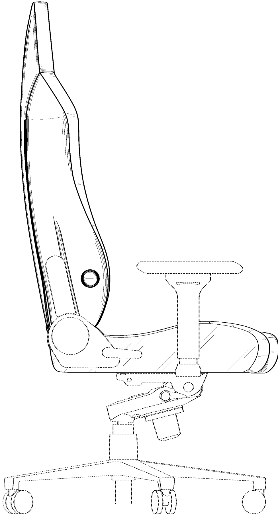
左側視圖
