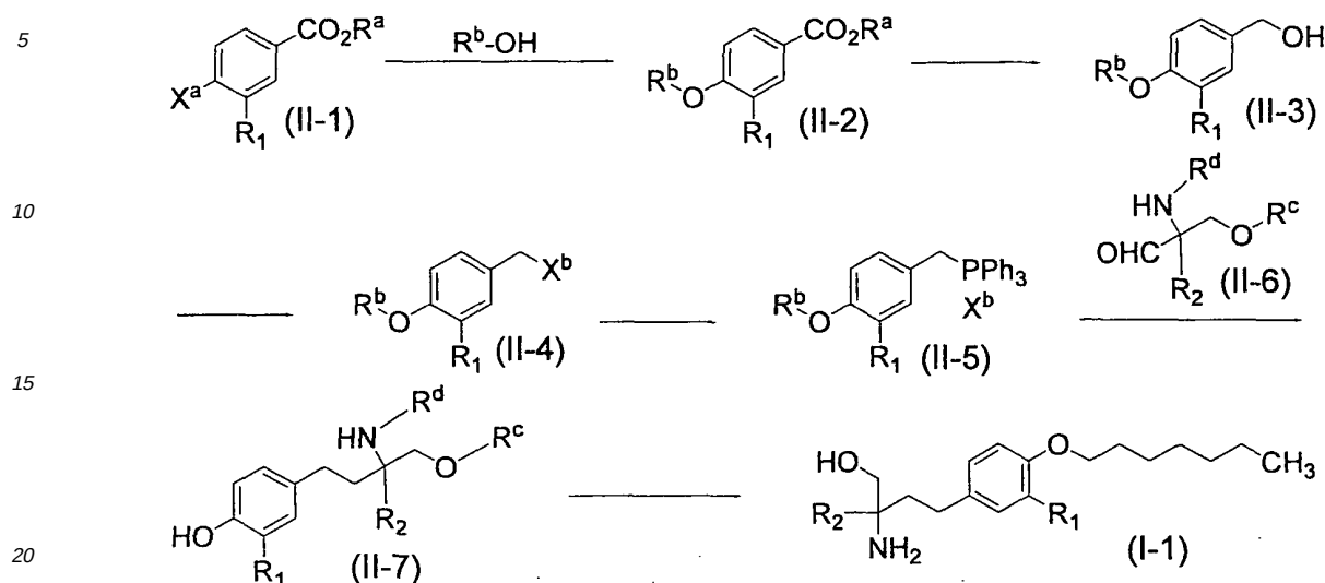
Schme (II)
