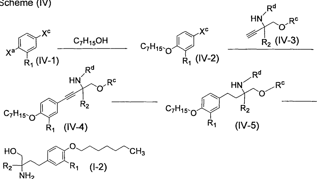
Scheme (IV)
