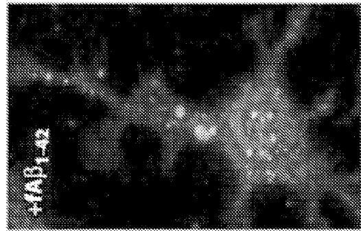
FIG. 5A WT
