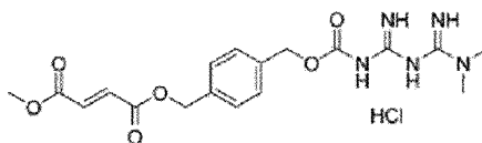
Verbindung 1
