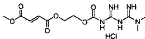
Verbindung 5
