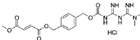
Composé 1
