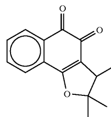
\alpha -DUNNIONE
