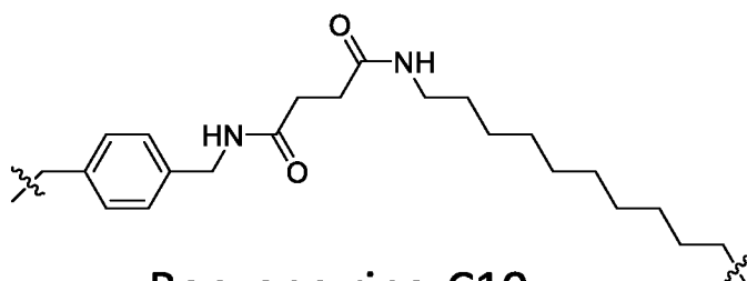
Benzene ring-C10
