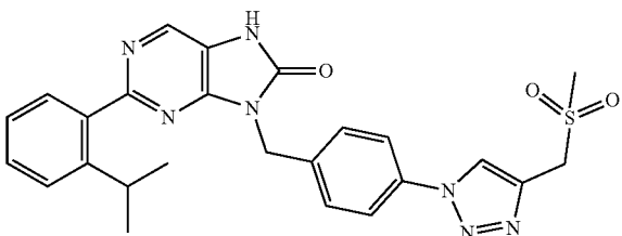
2-(2-isopropylphenyl)-9-(4-(4-((methylsulfonyl)methyl)-1H-1,2,3-triazol-1-yl)benzyl)-7,8-dihydro-8H-purin-8-one
