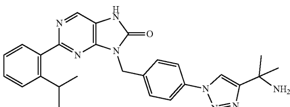
9-(4-(4-(2-aminopropan-2-yl)-1H-1,2,3-triazol-1-yl)benzyl)-2-(2-isopropylphenyl)-7,9-dihydro-8H-purin-8-one
