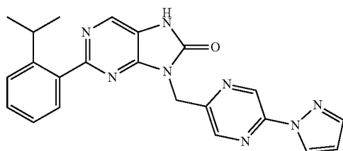
9-((5-(1H-pyrazol-1-yl)pyrazin-2-yl)methyl)-2-(2-isopropylphenyl)-7,9-dihydro-8H-purin-8-one
