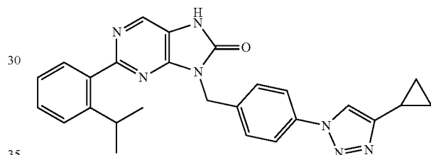
9-(4-(4-cyclopropyl)-1H-1,2,3-triazol-1-yl)benzyl)-2-(2-isopropylphenyl)-7,8-dihydro-8H-purin-8-one
