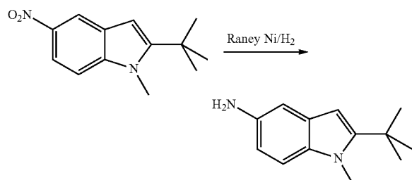
2-tert-Butyl-1-methyl-1H-indol-5-amine
