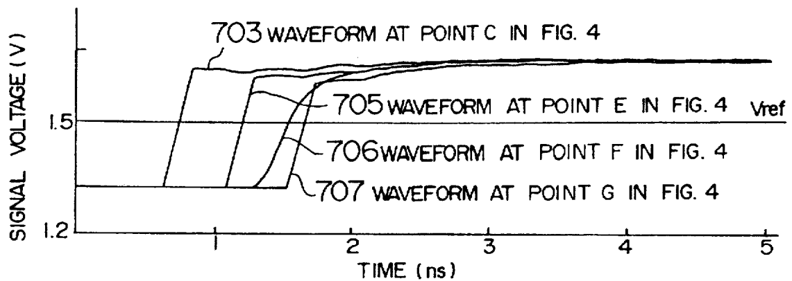
FIG. 18C
