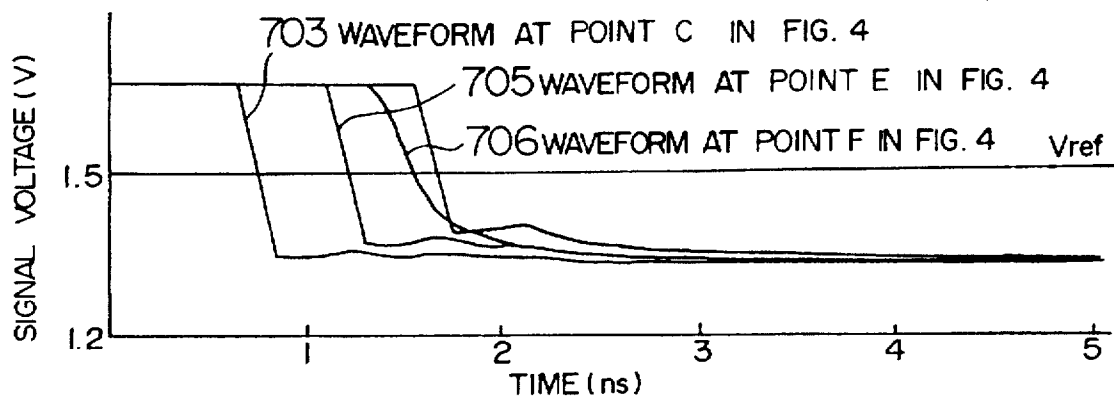
FIG. 19B
