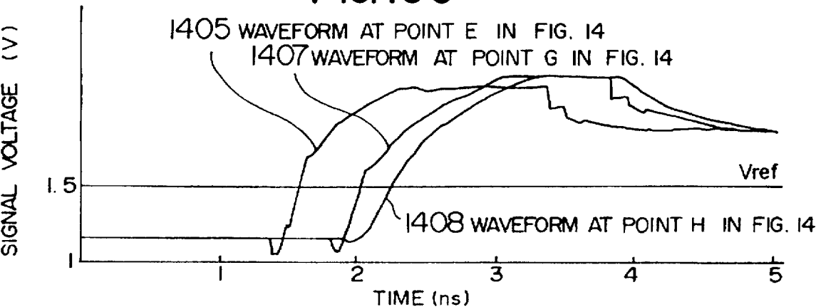
FIG. 16C
