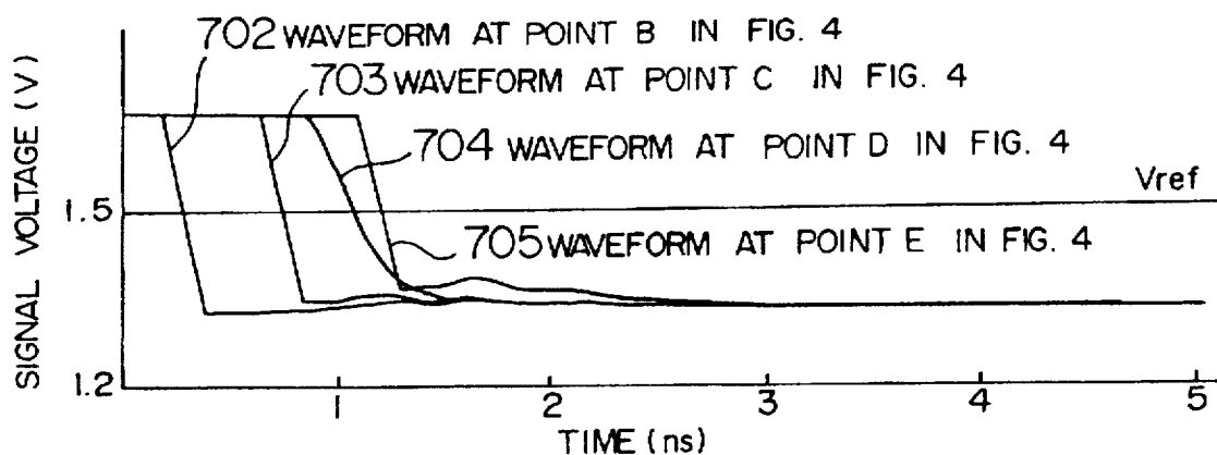
FIG. 19A
