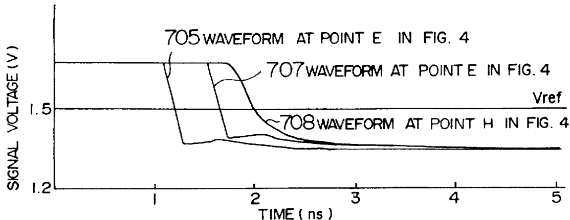
FIG. 19C
