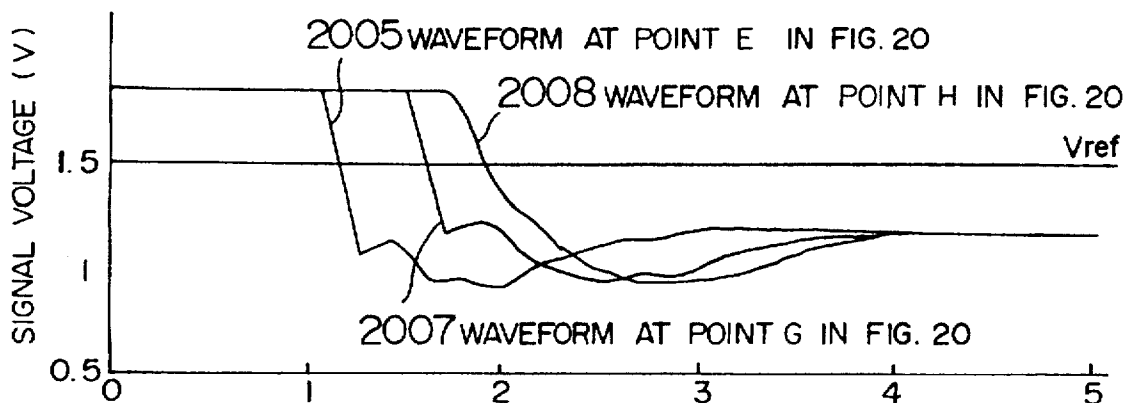
FIG. 23C
