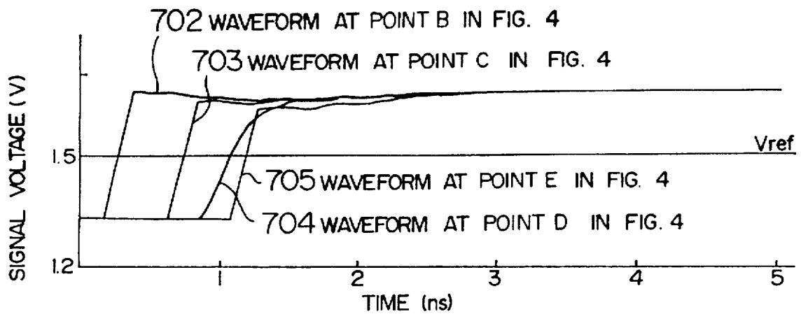
FIG. 18A
