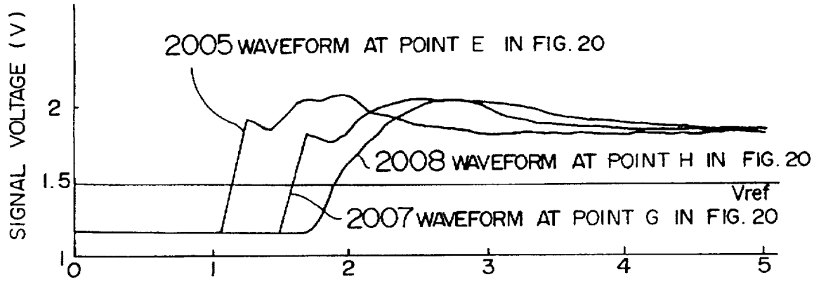
FIG. 22C
