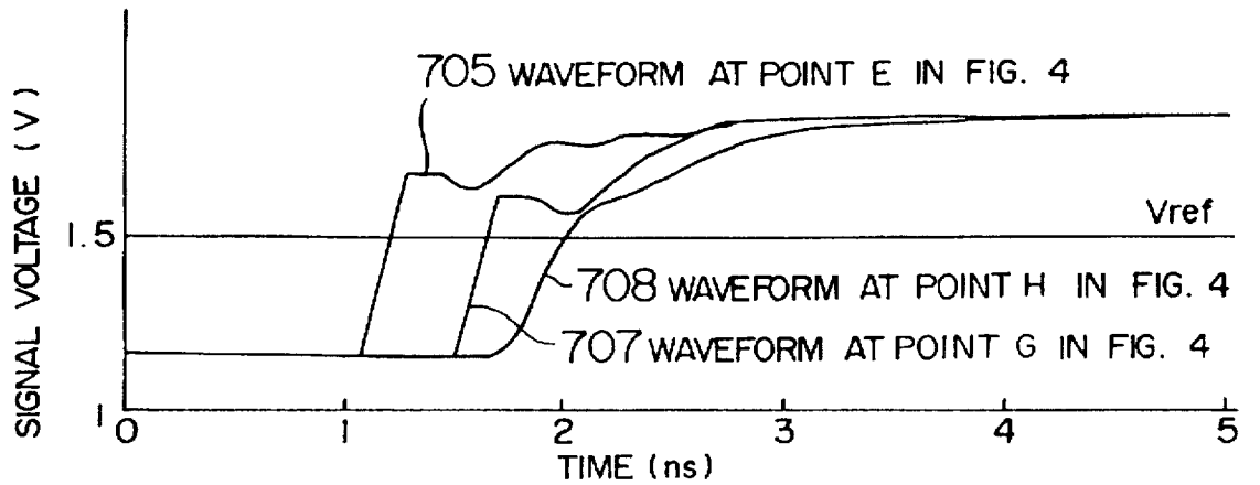
FIG. 7C
