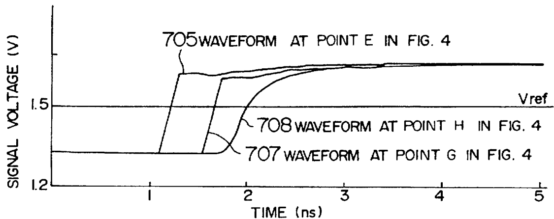
FIG. 18C
