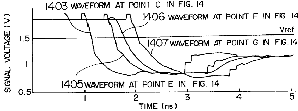
FIG. 17B
