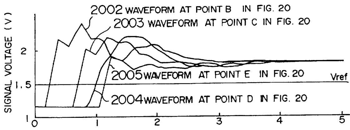
FIG. 22A
