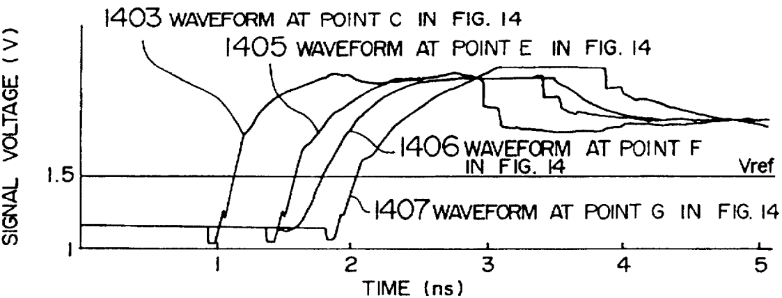
FIG. 16B
