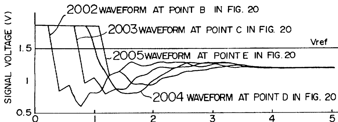
FIG. 23A
