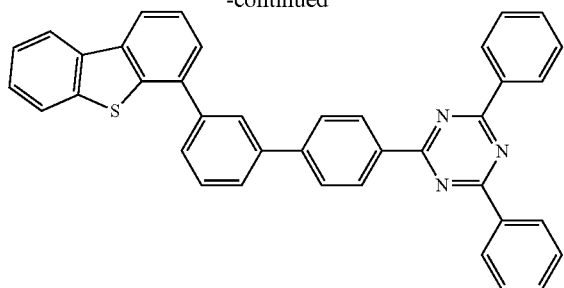
Compound D1
