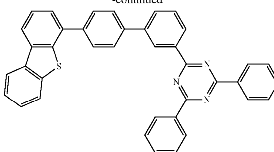
Compound D2
