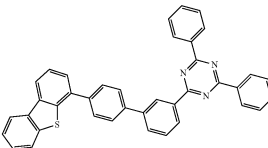
Compound D2
