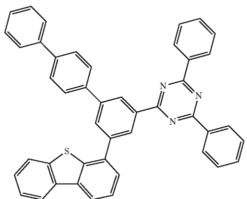
Compound A5
