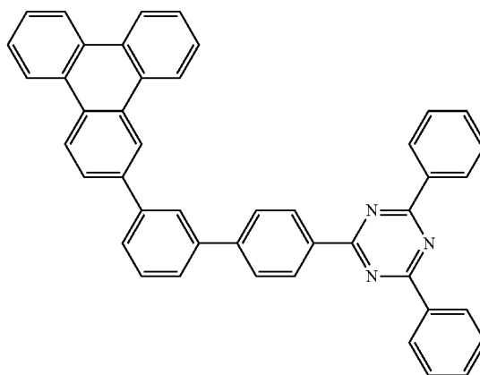
Compound D2
