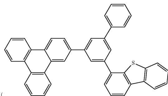
Compound E11
