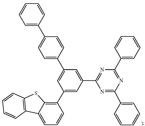
Compound A5
