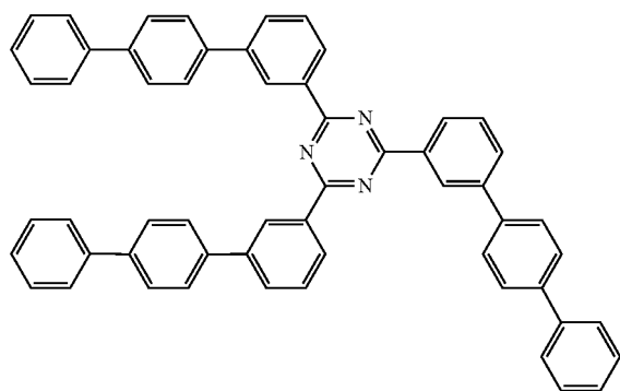
Compound F1
