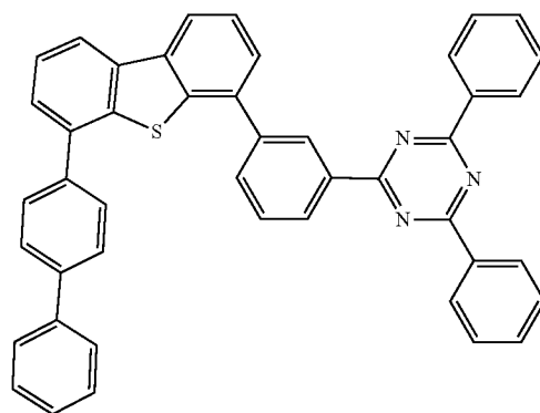
Compound E11
