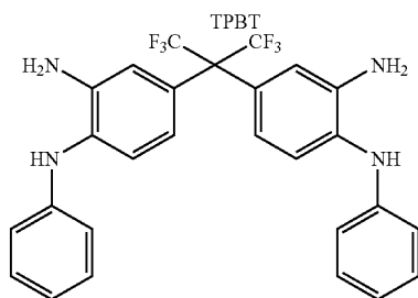
PhTA
