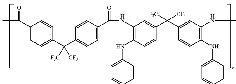
PA(HPBT-PhTA)
