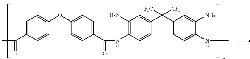
PA(OBBT-TA)
