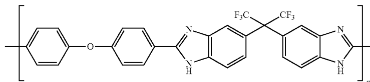
PBI(OBBT-TA)
