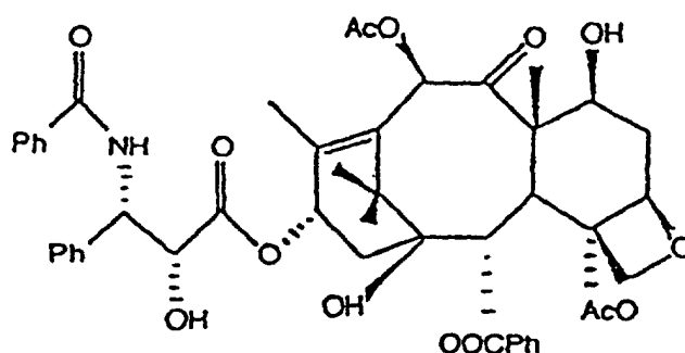
(a) Paclitaxel
