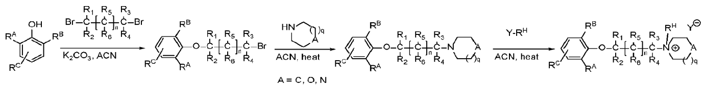
Scheme A:
