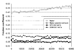
CC (a)各試料の摩擦係数
