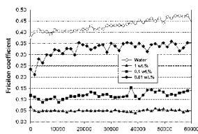
DD (b)SP1酸化グラフェンの摩擦係数
