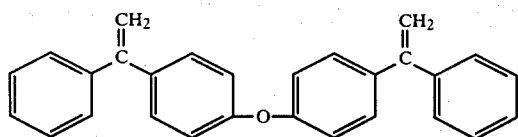
Bis [4-(1-phenylethenyl)phenylethenyl]phenyl ether
