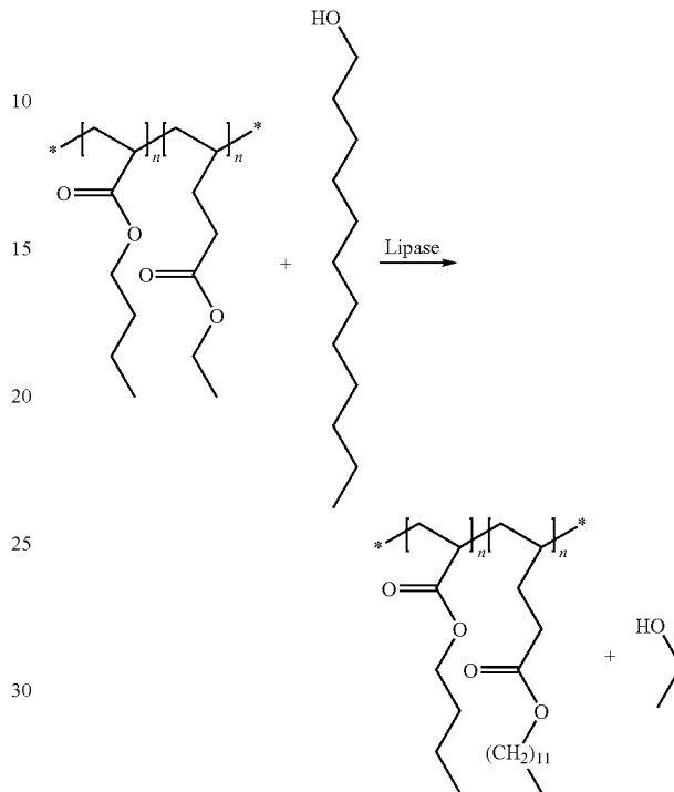
Scheme VI
