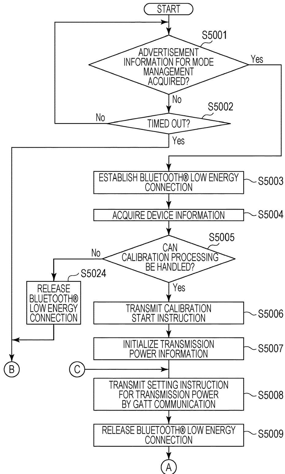
FIG. 5A
